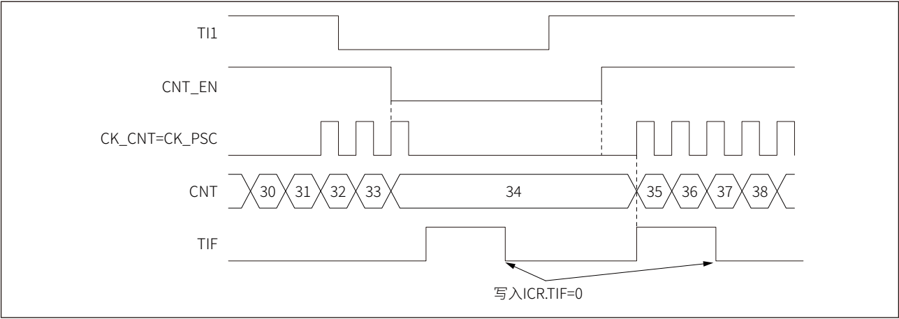
图 17-26 门控模式时序
