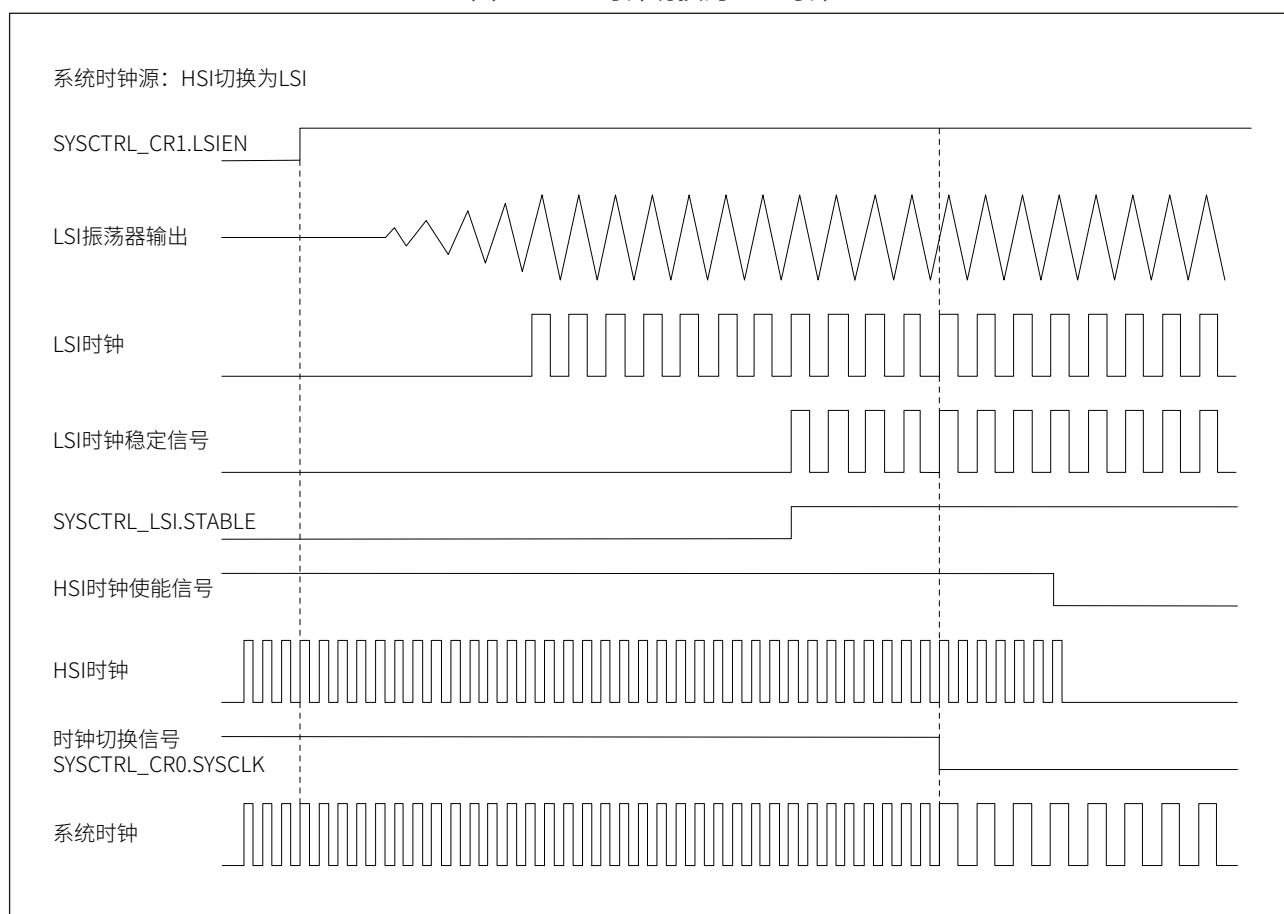
图 4-6 HSI 时钟切换为 LSI 时钟
