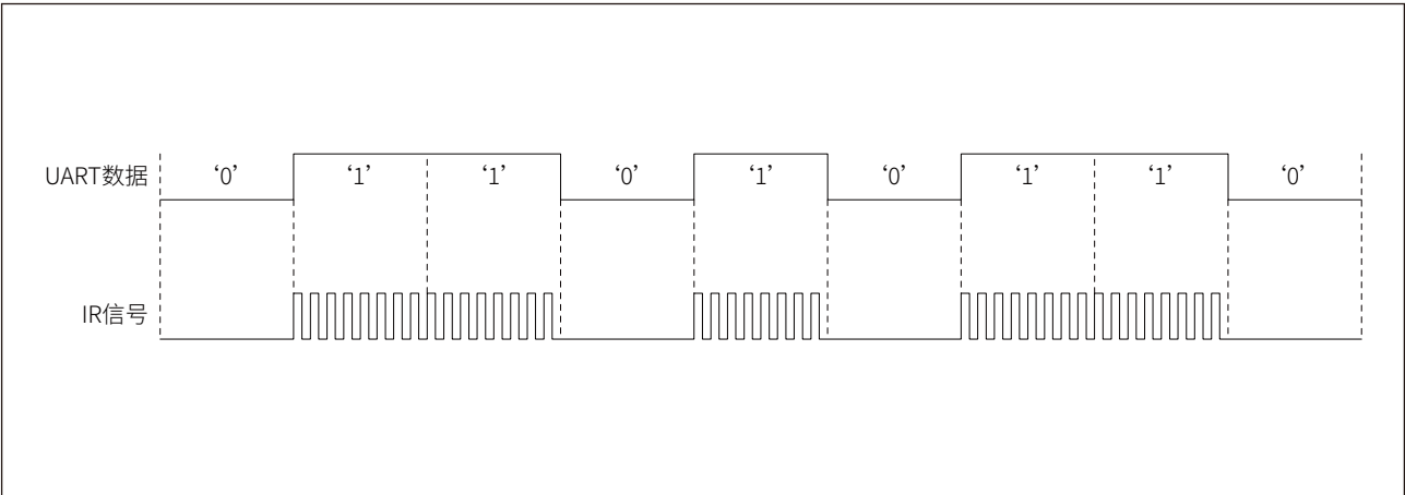
图 24-3 UART 调制方式
