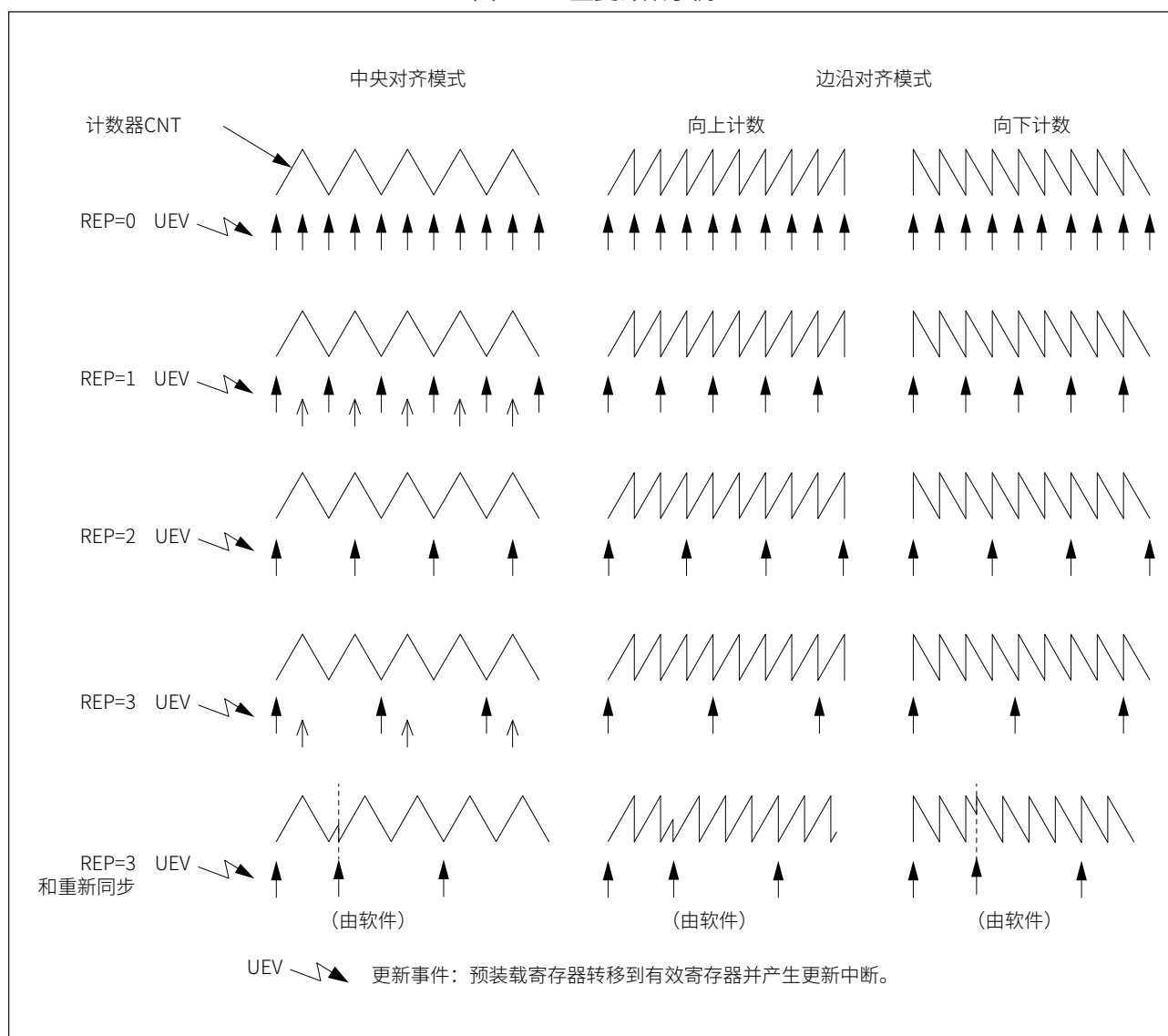
图 17-19 重复计数示例
