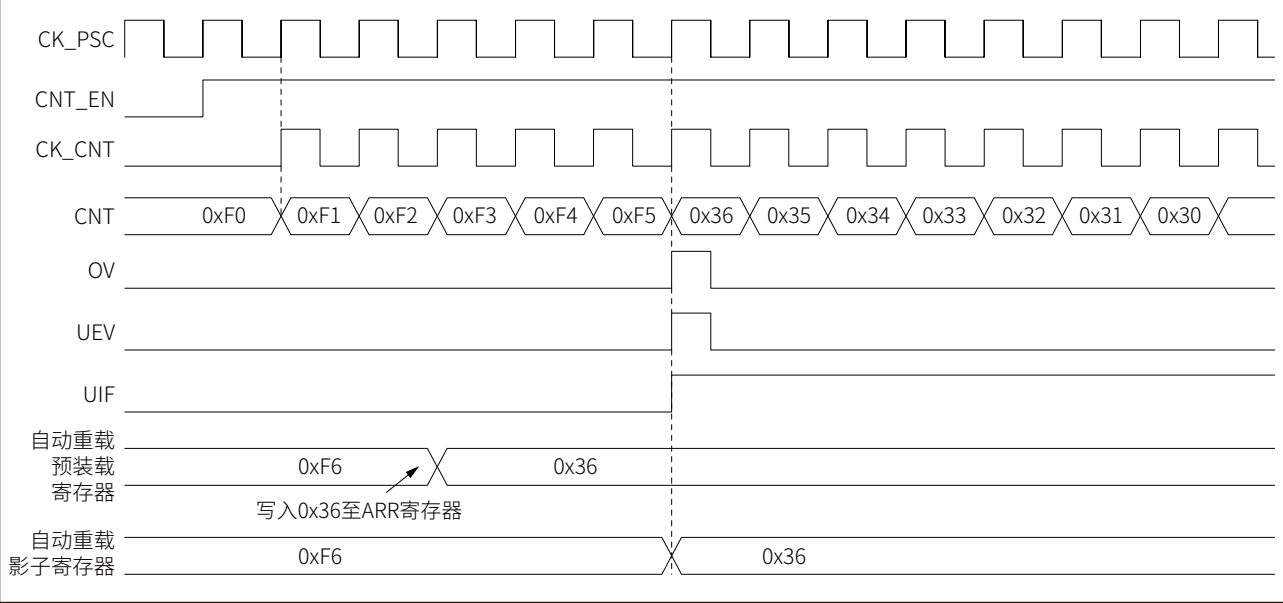
图 17-18 中心对齐模式，当重载缓存使能时的更新事件 (ATIM_CR1.ARPE=1)
