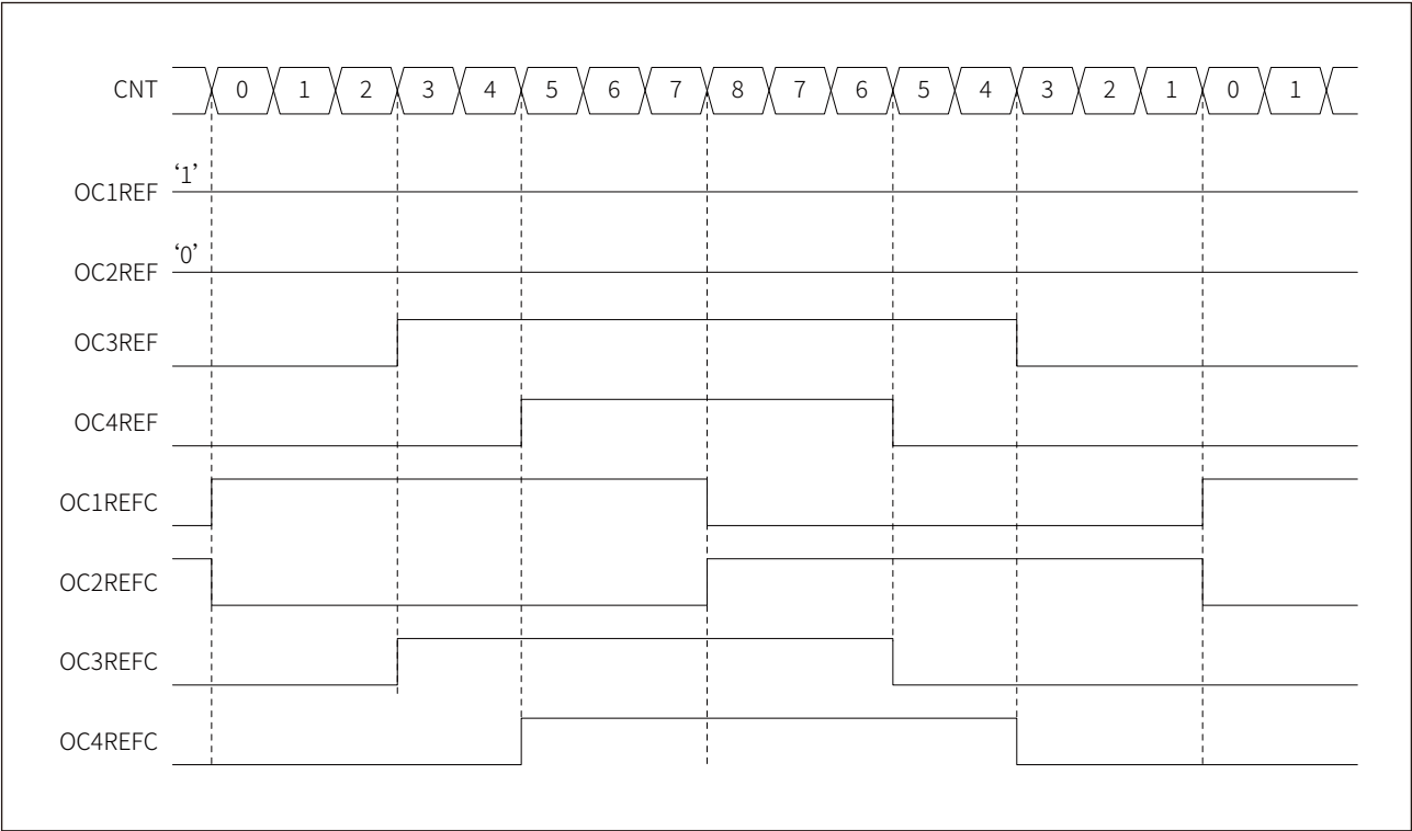
图 16-41 不对称 PWM 模式 2 示例
