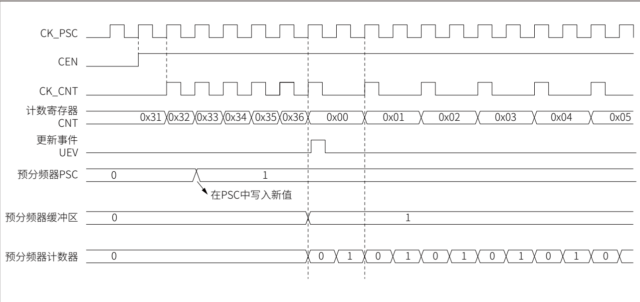
图 16-2 预分频器分频由 1 变为 2 时的时序图
