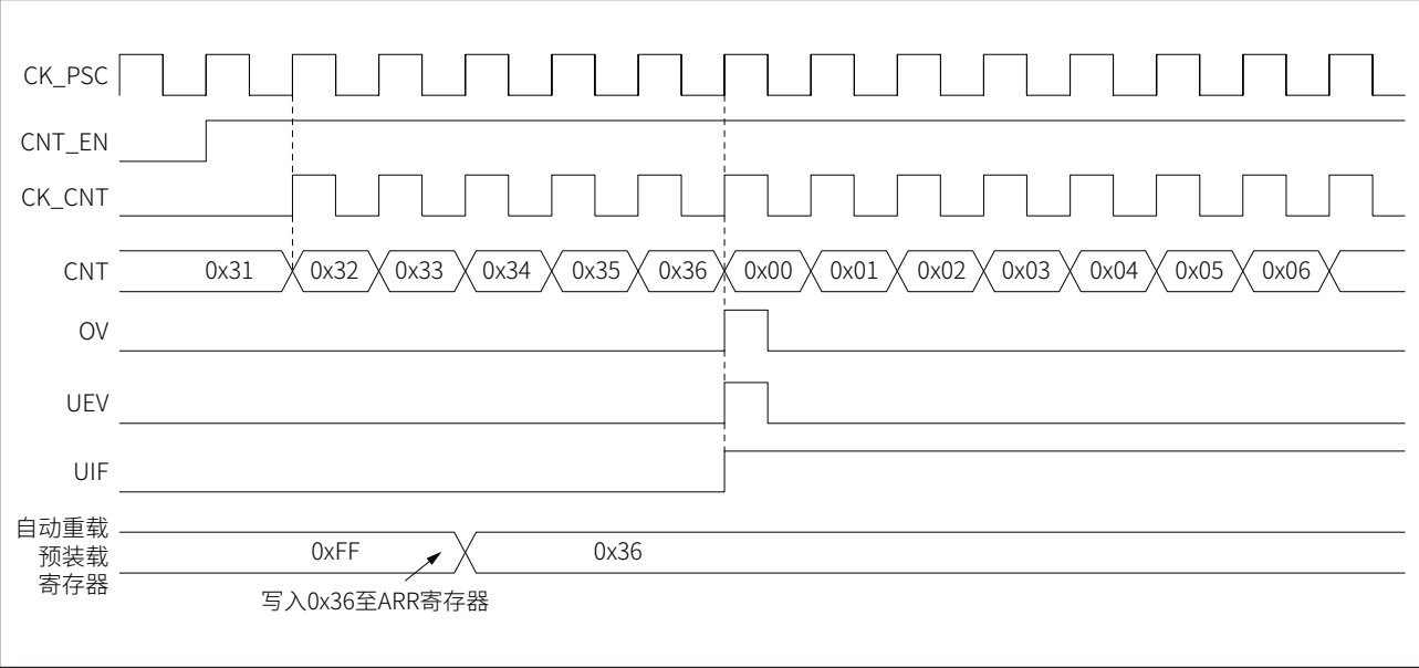
图 16-8 递增计数，当重载缓存使能时的更新事件 (GTIMx_CR1.ARPE=1)
