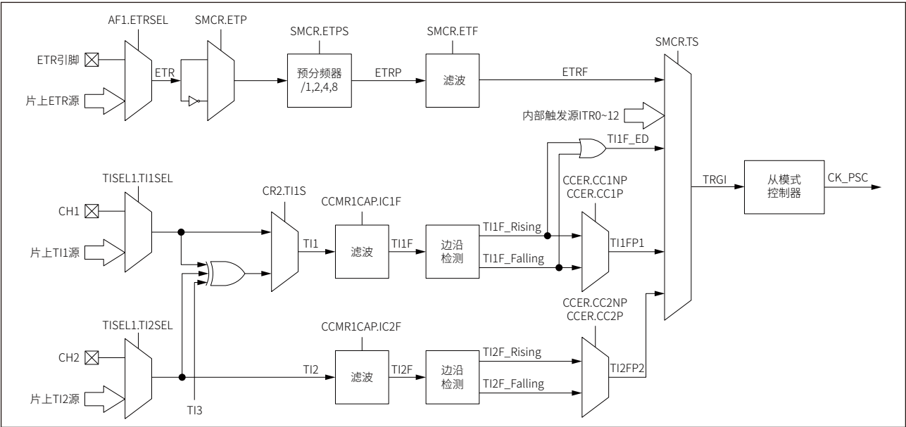
图 17-22 外部时钟模式 1 连接图
