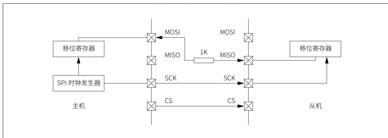
图 22-7 单线半双工模式
