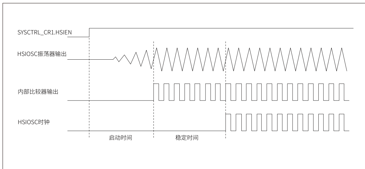
图 4-4 HSIOSC 时钟启动过程
