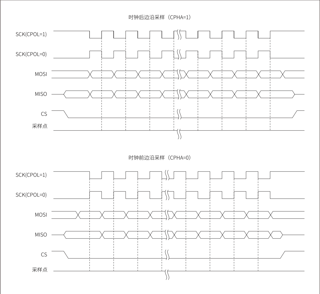
图 22-2 SPI 通信时序
