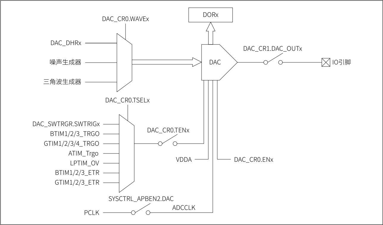
图 26-1 DAC功能框图
