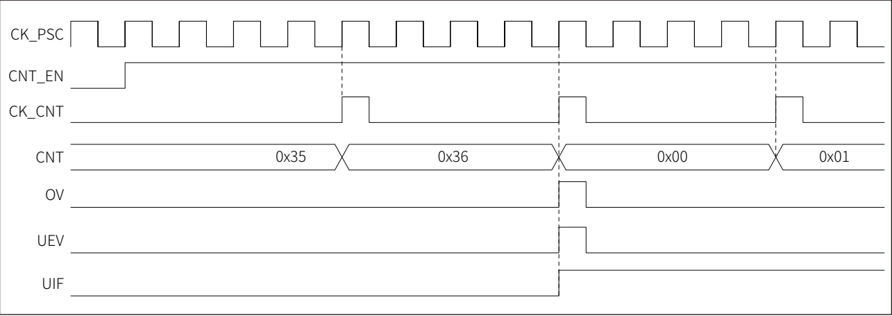
图 16-6 递增计数，内部时钟分频因子为 N
