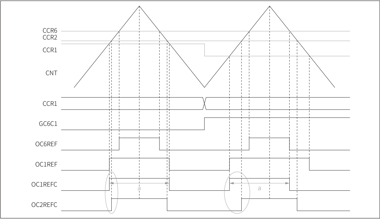
图 17-45 移相 PWM 模式 6 示例
