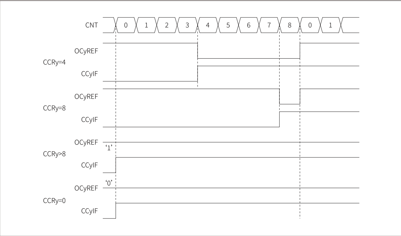
图 17-37 PWM 模式 1，边沿对齐模式，递增计数
