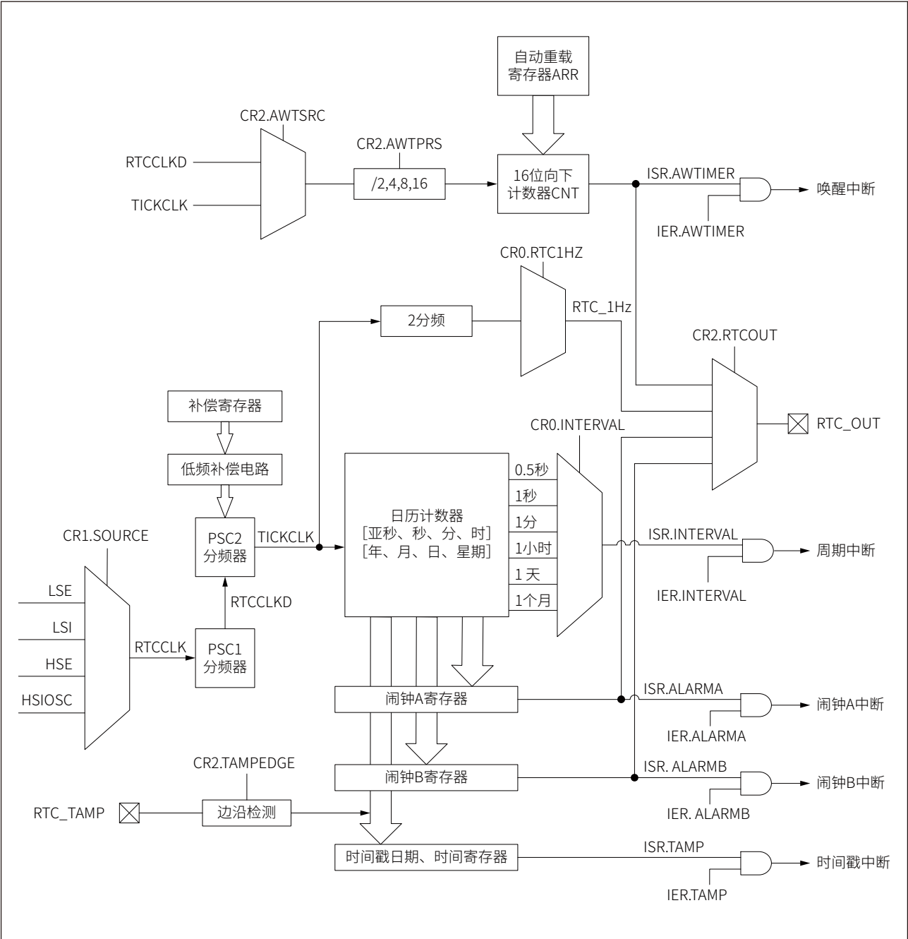
图 13-1 RTC 功能框图
