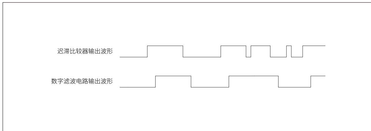
图 28-3 LVD 滤波输出
