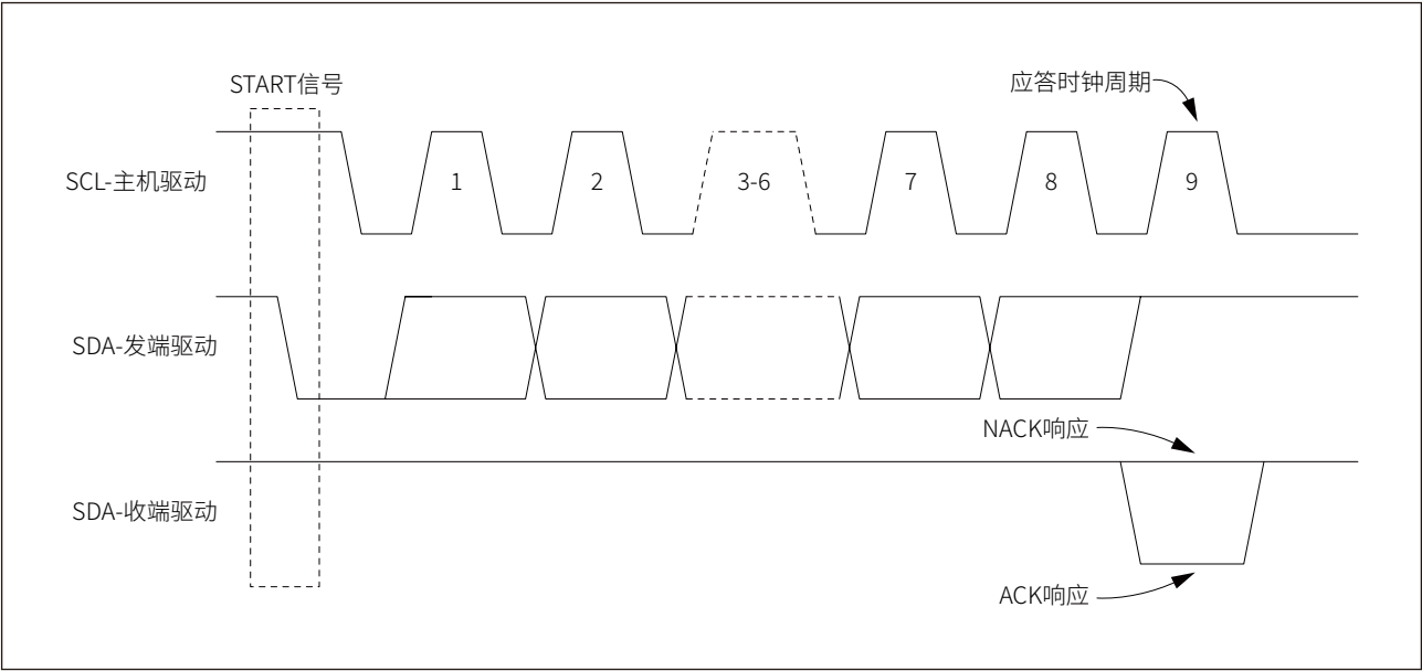
图 23-4 传输应答
