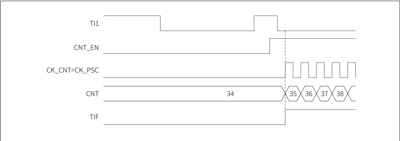
图 16-26 触发模式时序
