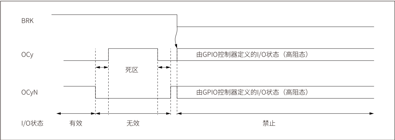
图 17-50 响应刹车事件 BRK 时的输出行为 (OSSI=0)
