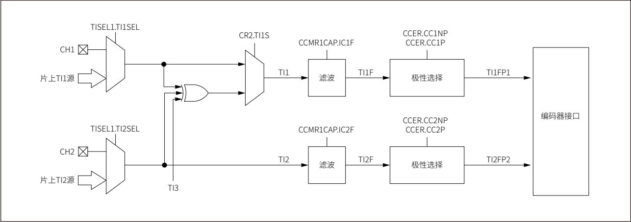
图 17-28 编码器模式框图
