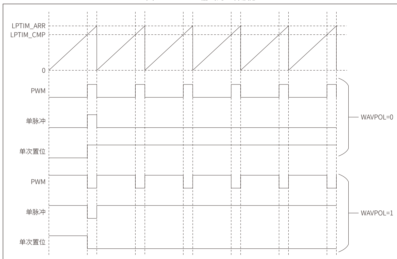
图 15-6 LPTIM 输出的三种波形
