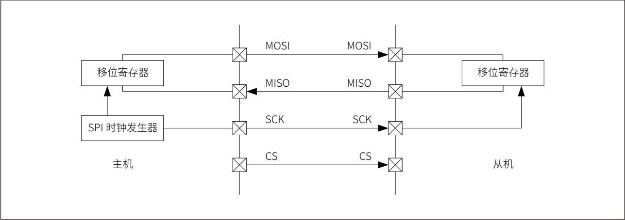
图 22-4 全双工通信模式
