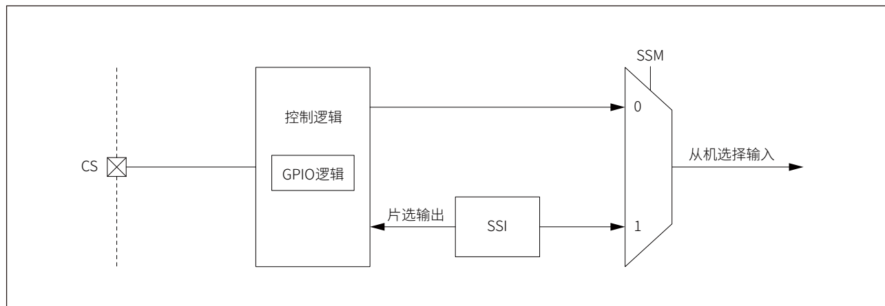
图 22-3 从机选择引脚管理
