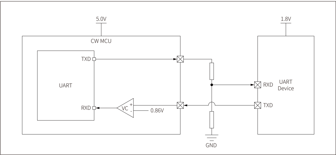
图 21-11 不同电压器件通信示意图
