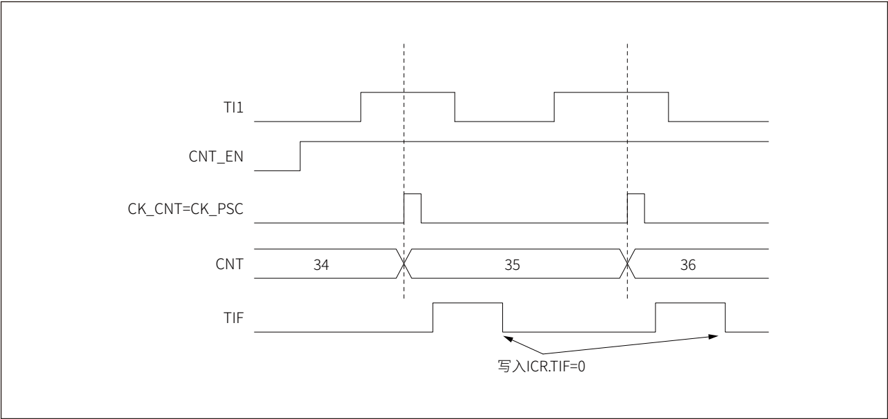
图 16-22 外部时钟模式 1 时序示例
