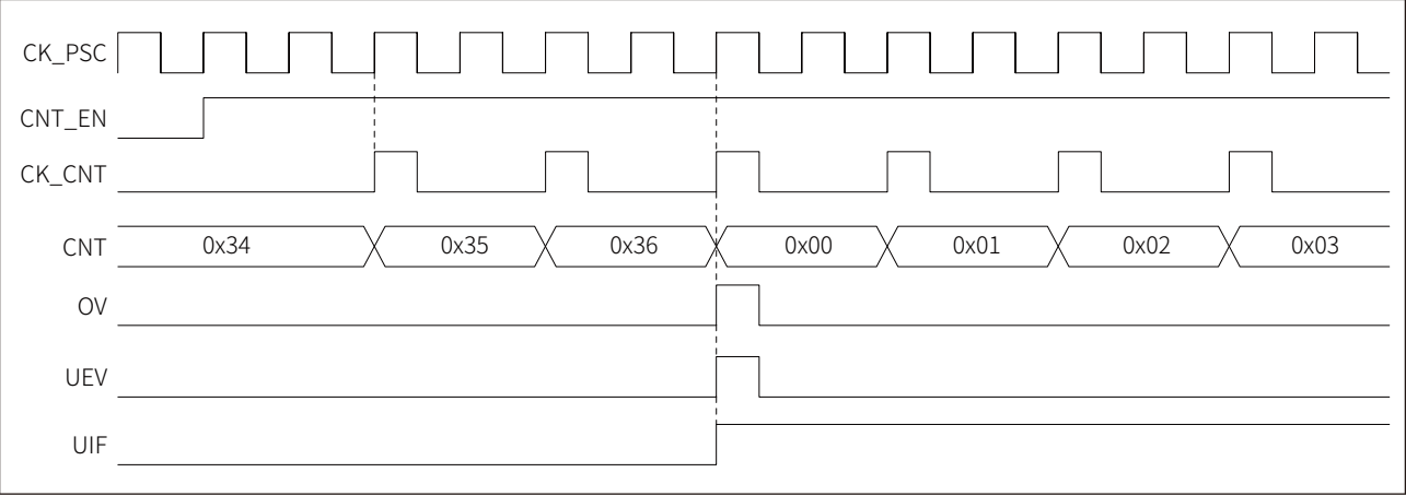
图 16-5 递增计数，内部时钟分频因子为 4
