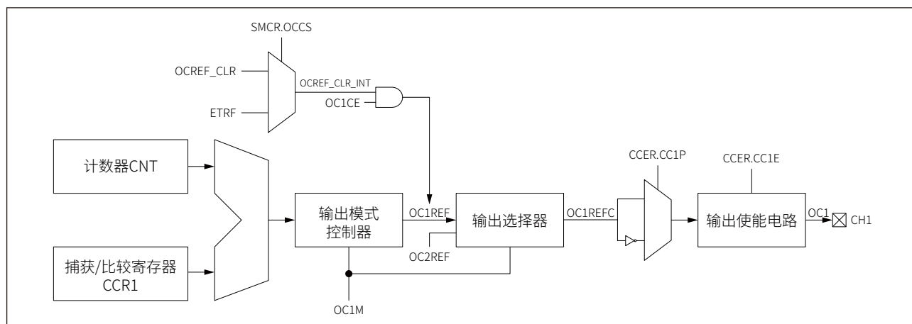
图 16-20 输出比较 1 通道
