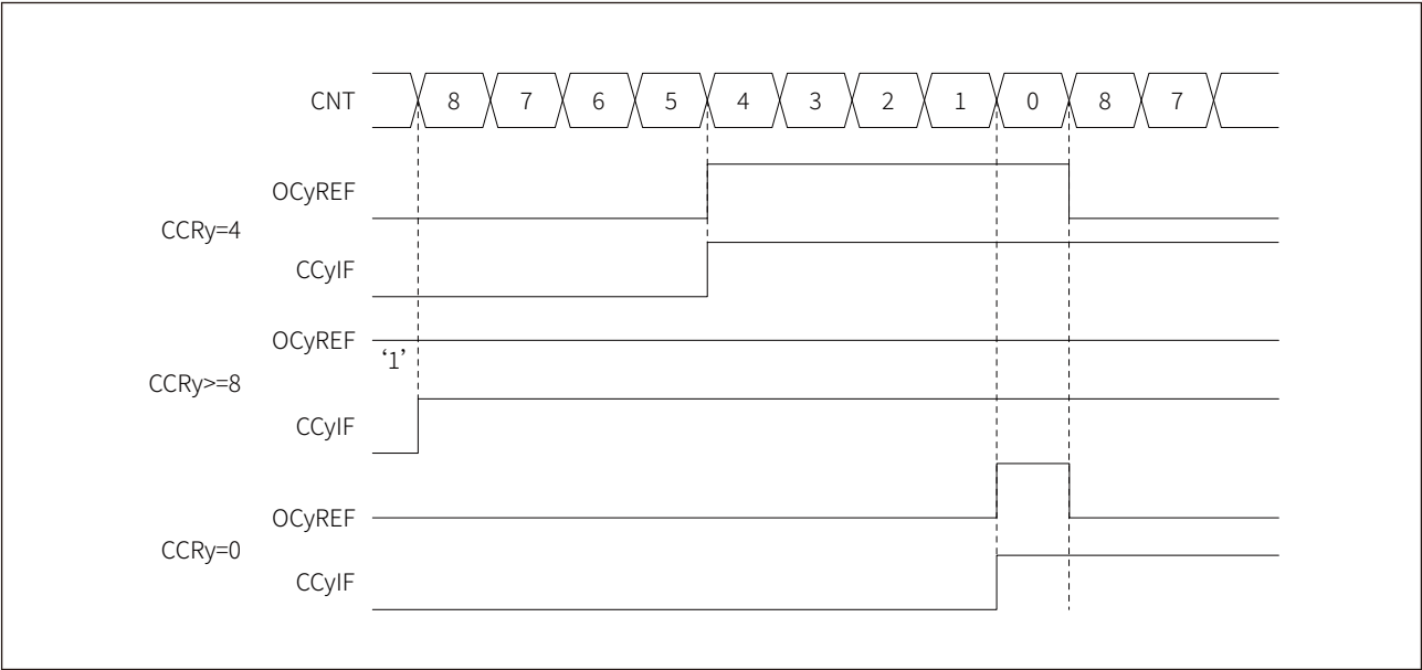
图 17-39 PWM 模式 1，中心对齐模式
