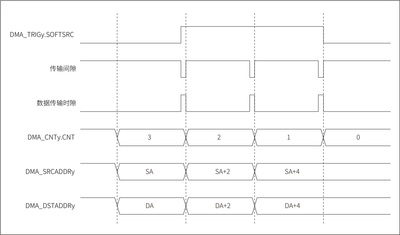
图 8-2 软件触发BLOCK传输模式
