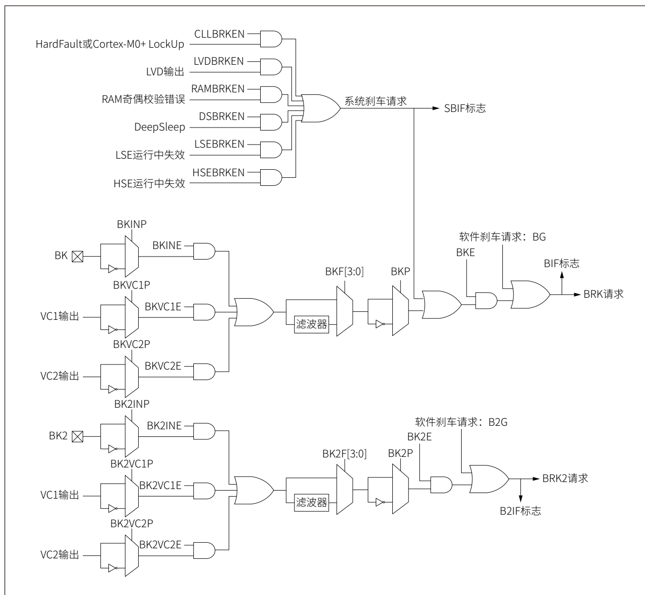
图 17-48 刹车和刹车 2 电路
