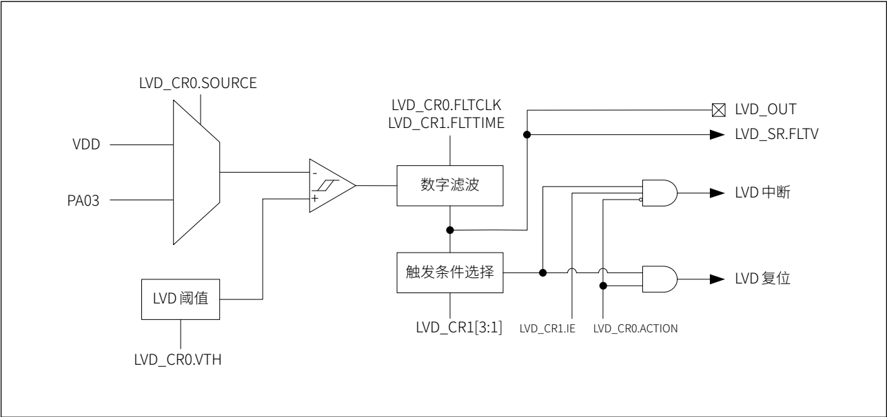
图 28-1 LVD 功能框图
