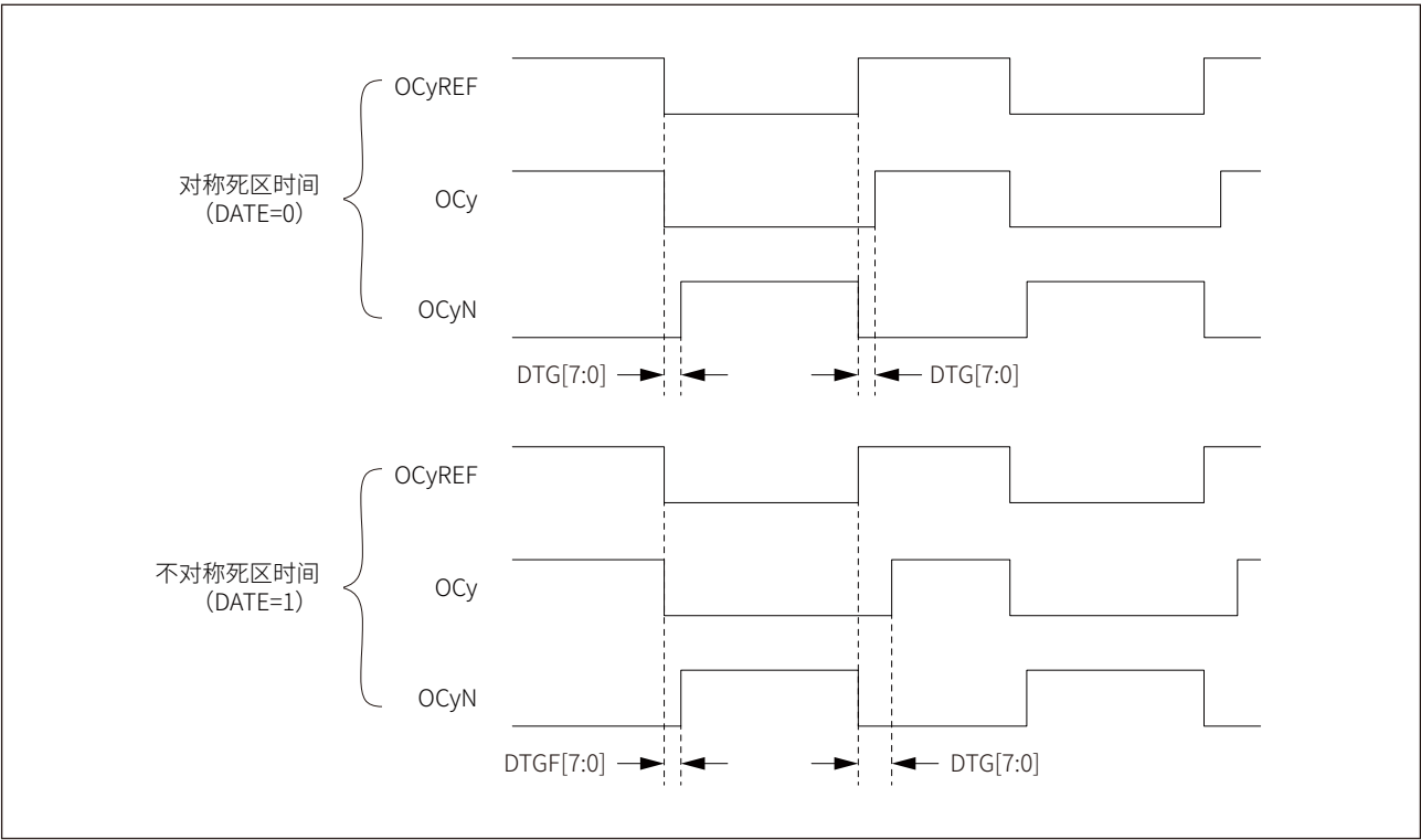
图 17-47 带死区插入的互补 PWM 输出波形
