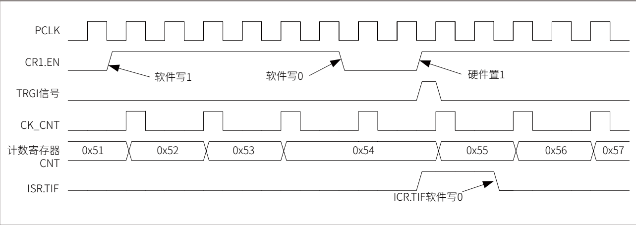
图 14-8 触发启动模式时序图
