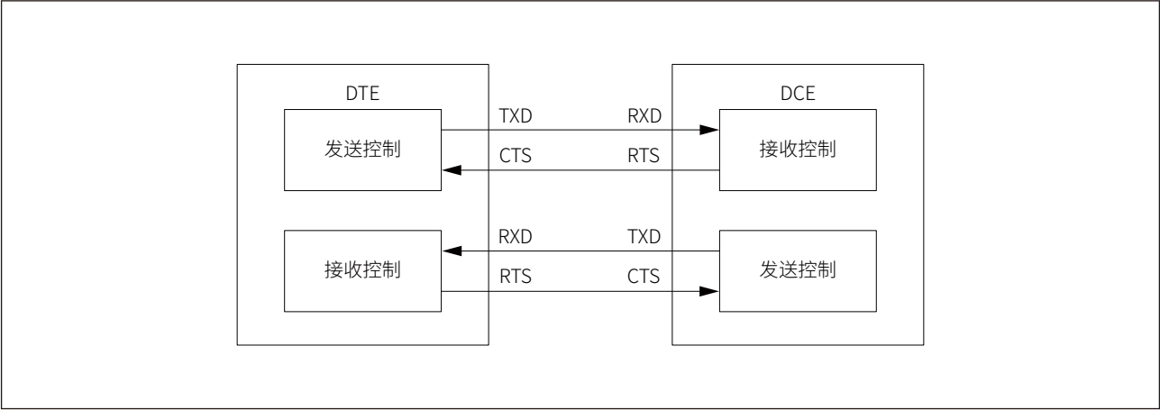
图 21-7 硬件流控示意图
