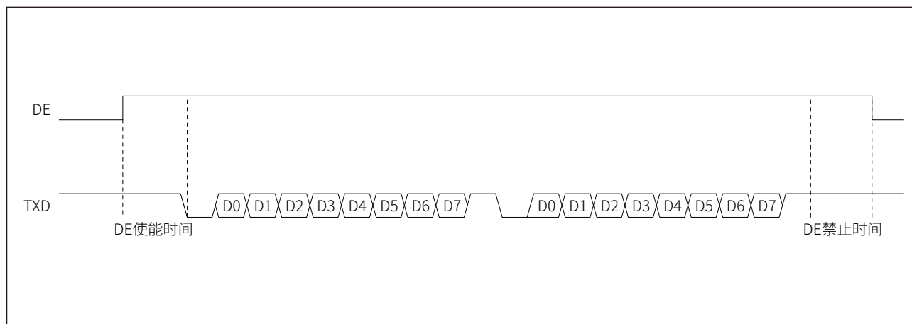
图 21-10 驱动器使能时序
