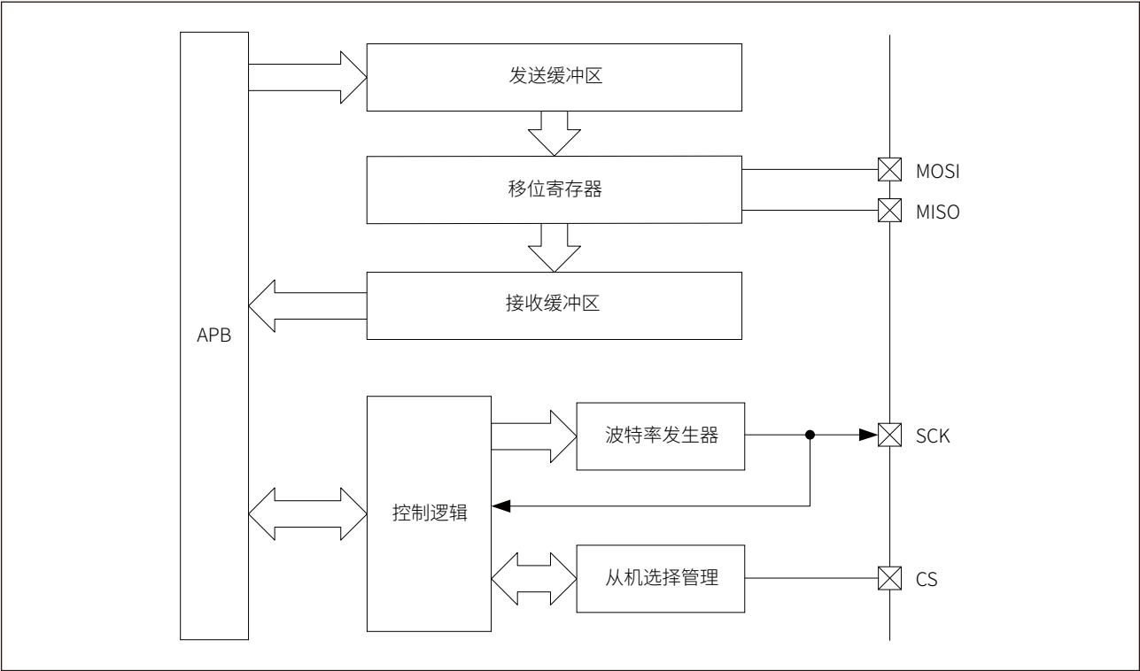
图 22-1 SPI 功能框图
