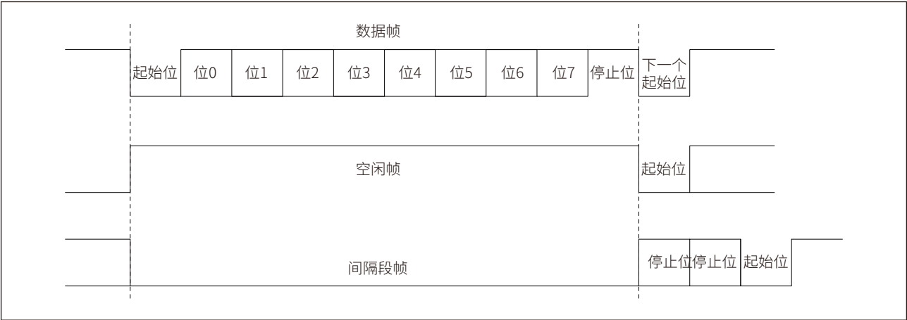
图 21-5 间隔段帧和空闲帧时序
