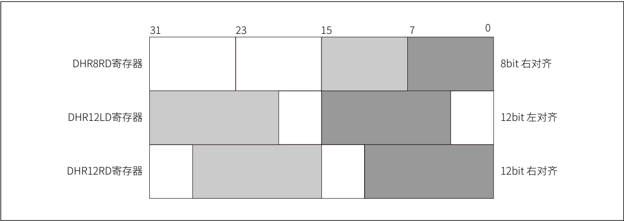
图 26-3 双通道寄存器配置格式
