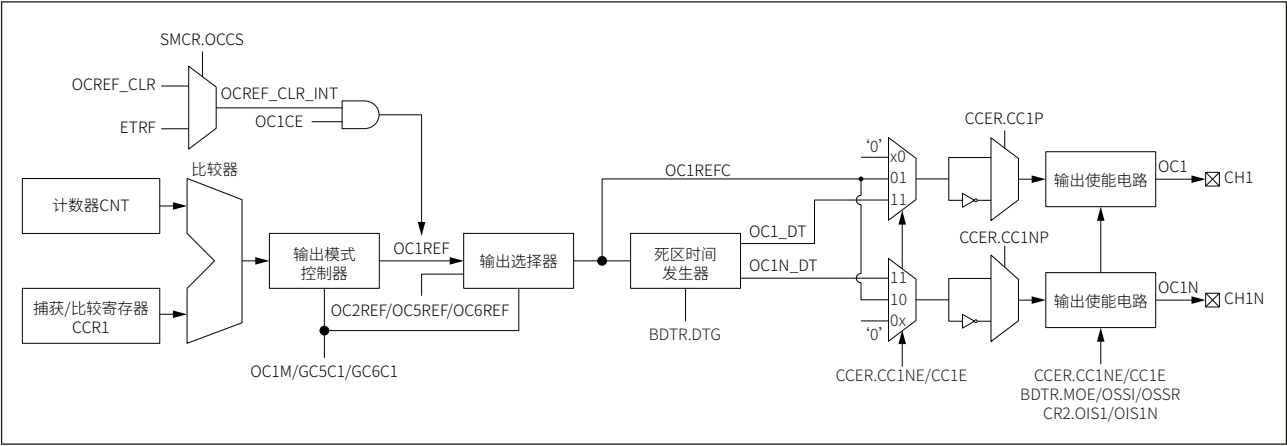
图 17-21 输出比较 1 通道
