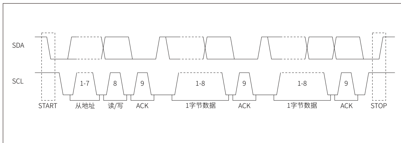
图 23-1 I2C 协议帧
