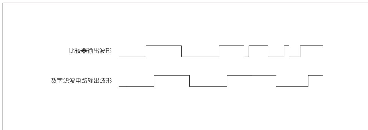
图 27-2 VC 滤波响应时间
