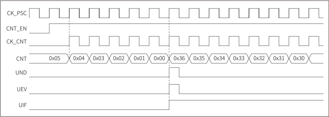
图 17-10 递减计数，内部时钟分频因子为 2
