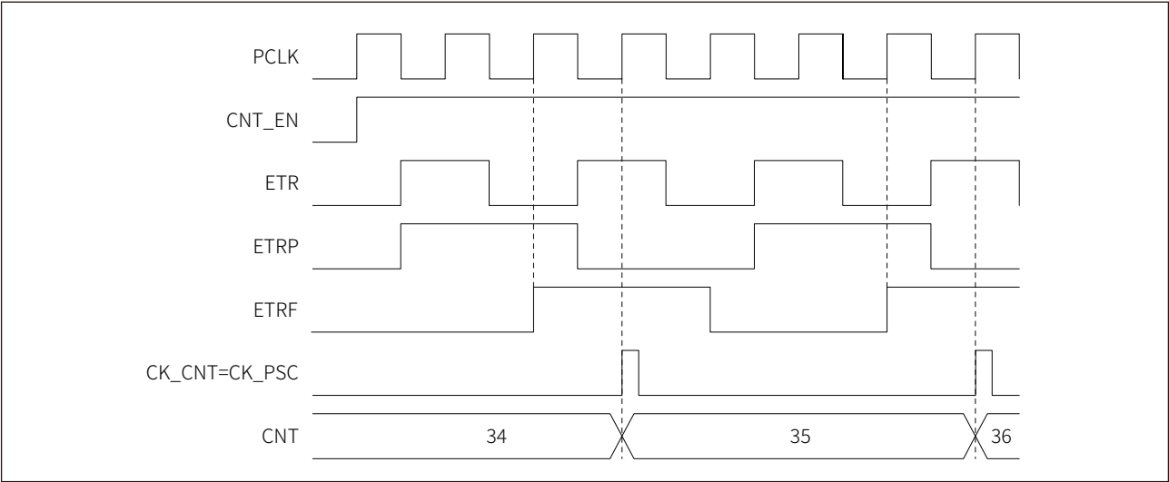
图 16-23 外部时钟模式 2 时序示例
