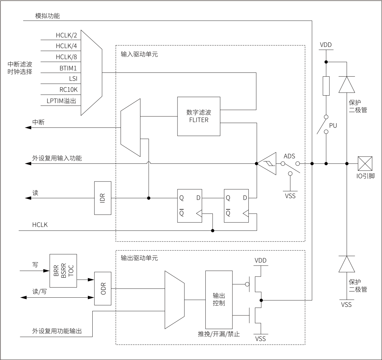
图 9-1 GPIO 功能框图
