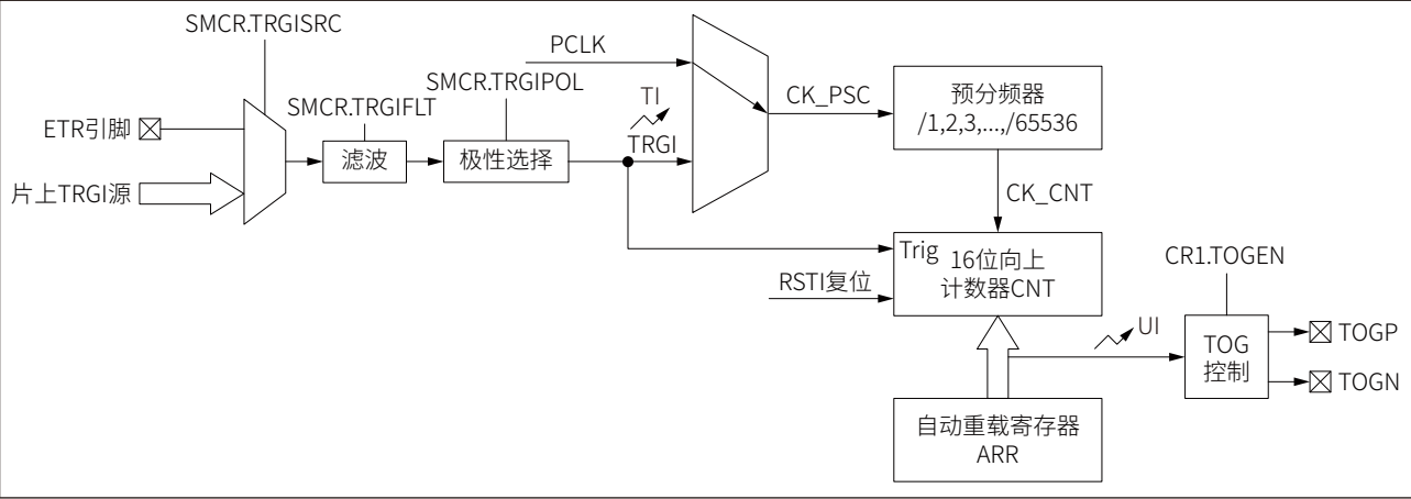
图 14-7 触发启动模式框图
