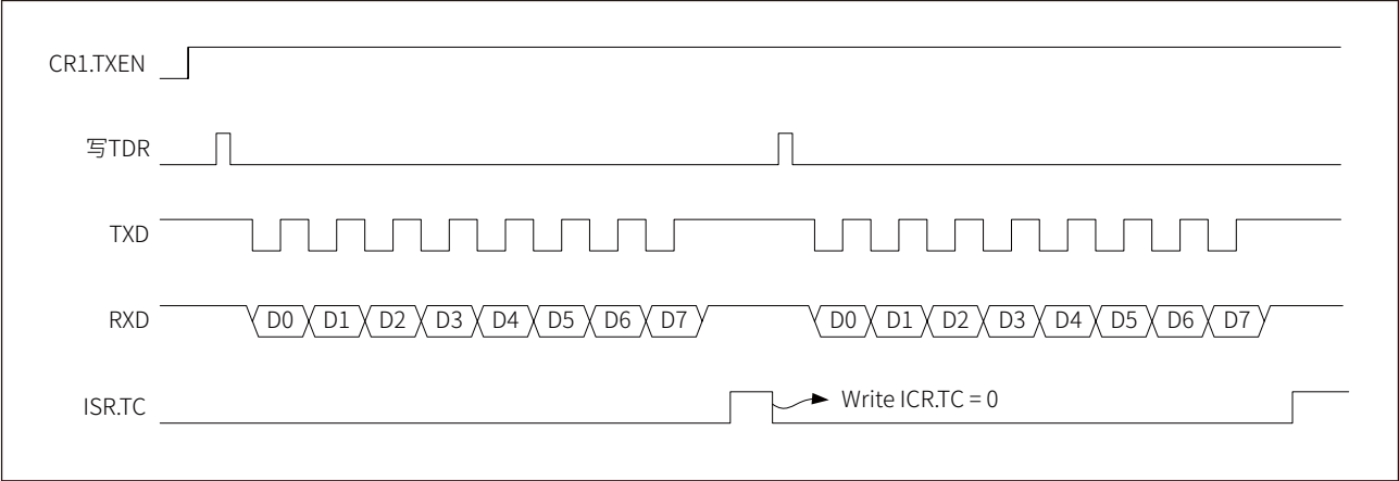
图 21-2 同步半双工模式发送时序（发送两个字节数据）
