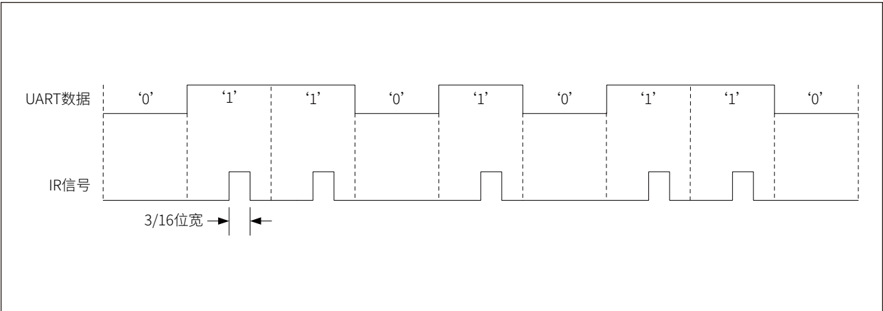
图 24-4 高速 UART 调制方式
