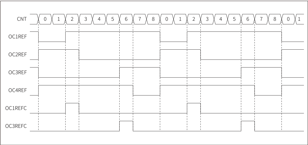
图 17-43 组合 PWM 模式 2 示例
