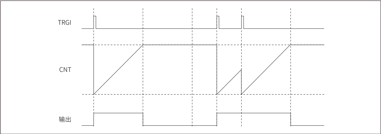
图 16-44 可再触发单脉冲模式 2 示例
