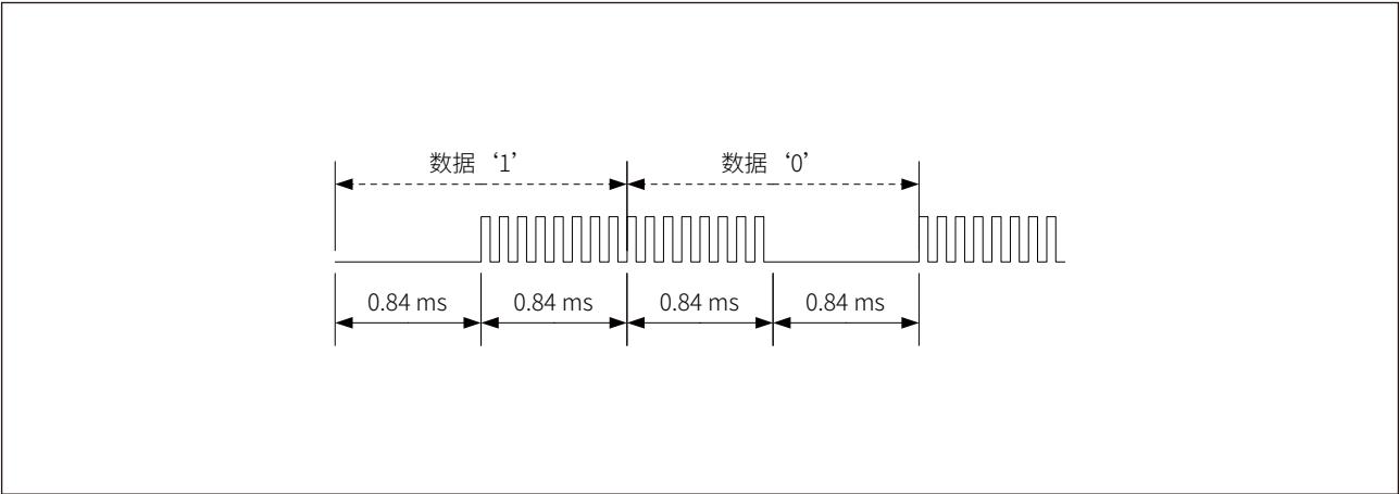
图 24-2 PPM 调制方式
