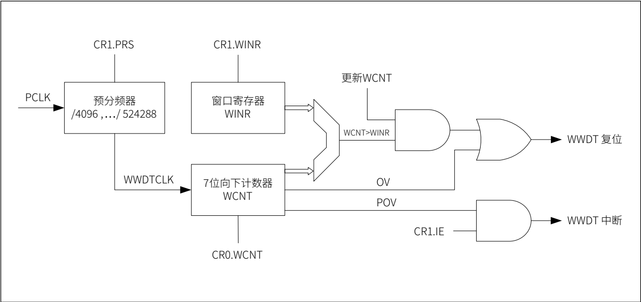
图 20-1 WWDT 功能框图
