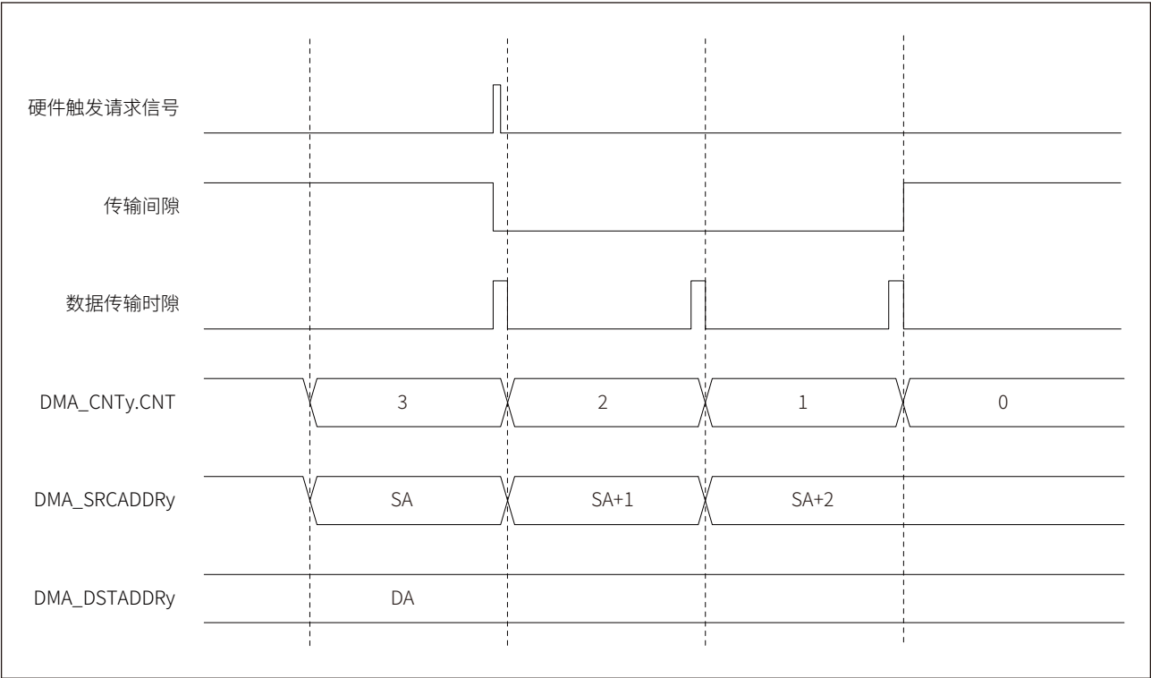
图 8-5 硬件触发 BULK 传输模式
