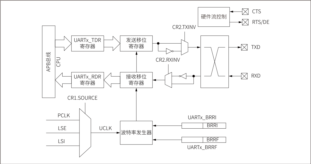
图 21-1 UART 功能框图
