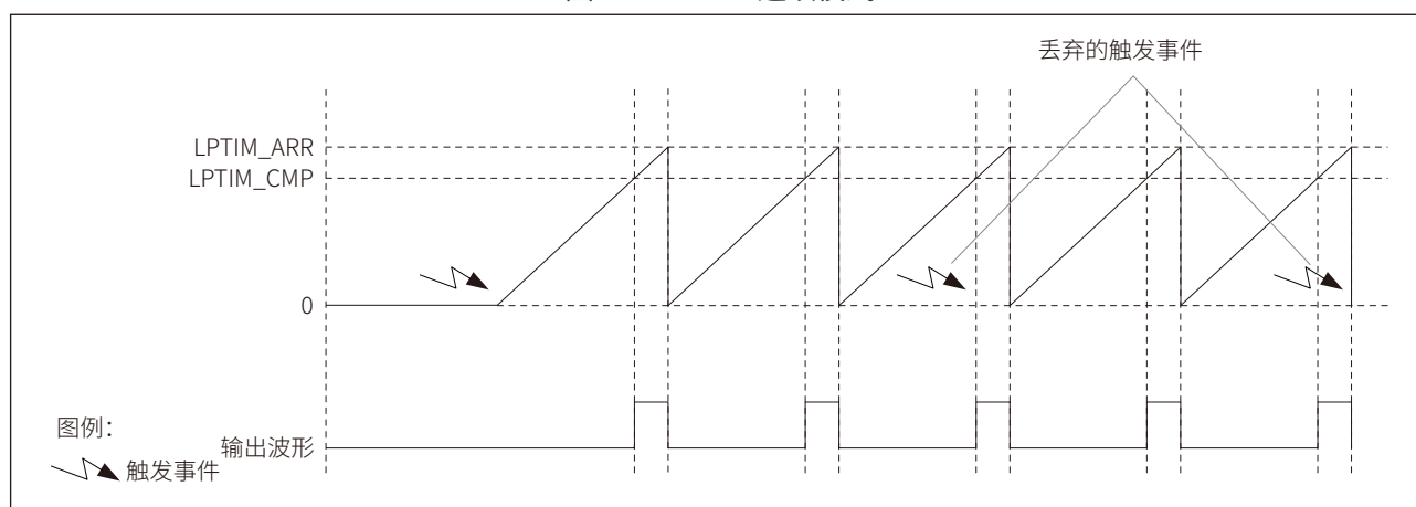
图 15-5 LPTIM 连续模式
