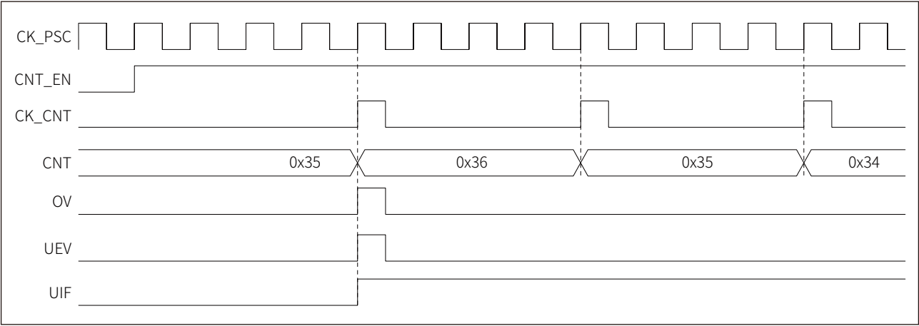
图 16-16 中心对齐模式，内部时钟分频因子为 N
