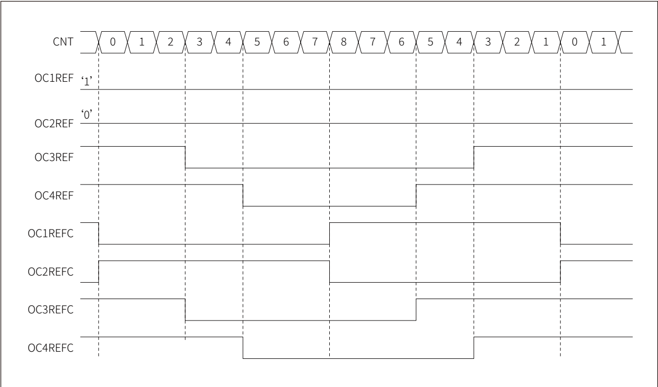
图 17-40 不对称 PWM 模式 1 示例
