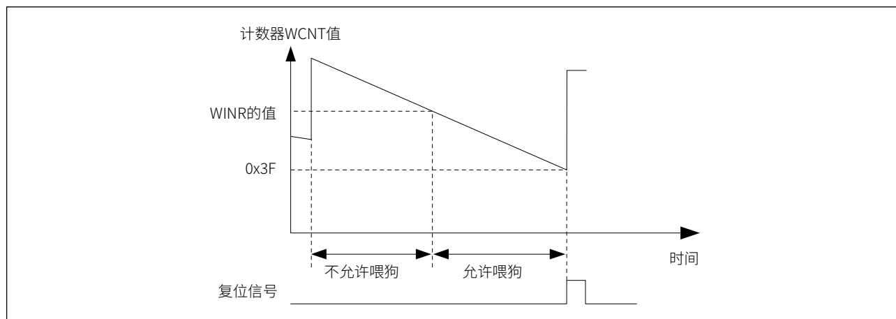
图 20-2 窗口看门狗的刷新（喂狗）时机
