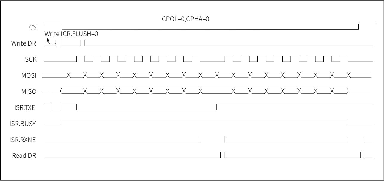
图 22-6 全双工模式下从机收发时序（两个字节）
