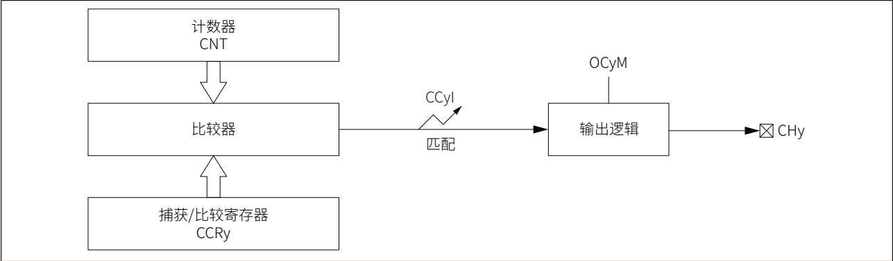
图 16-35 输出比较模式框图
