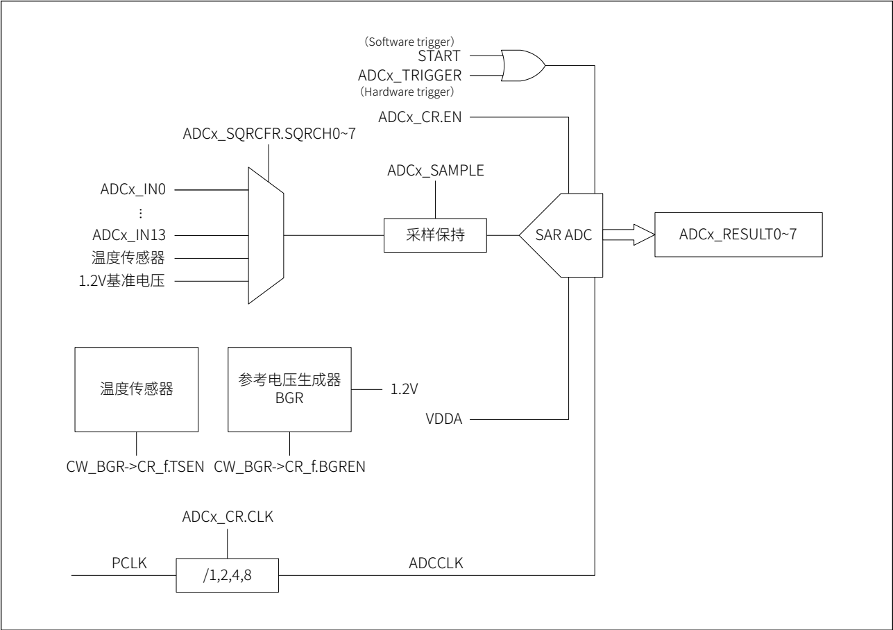
图 25-1 ADC 功能框图
