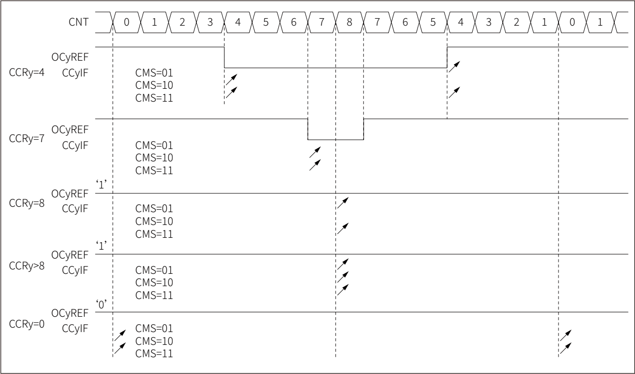
图 17-39 PWM 模式 1，中心对齐模式
