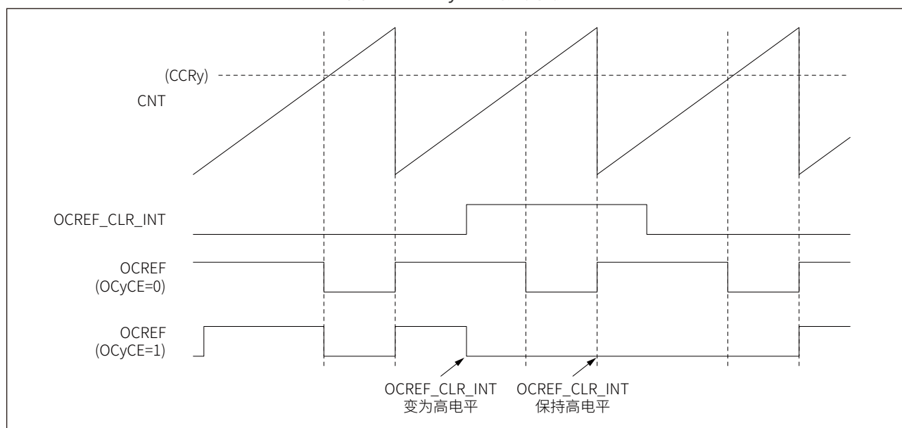
图 16-45 OCyREF 清零示例
