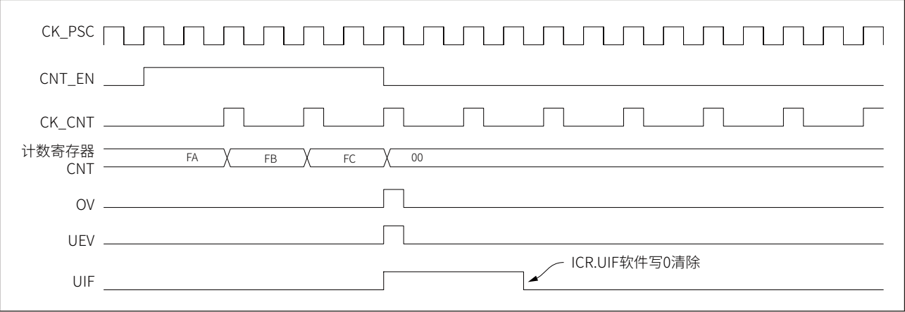
图 14-2 单次计数模式示例
