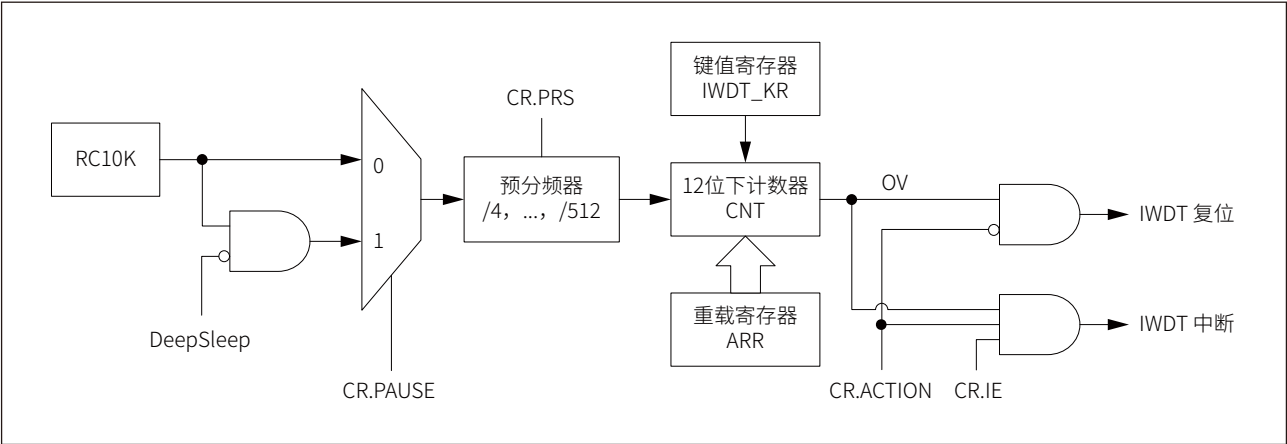
图 19-1 IWDT 功能框图
