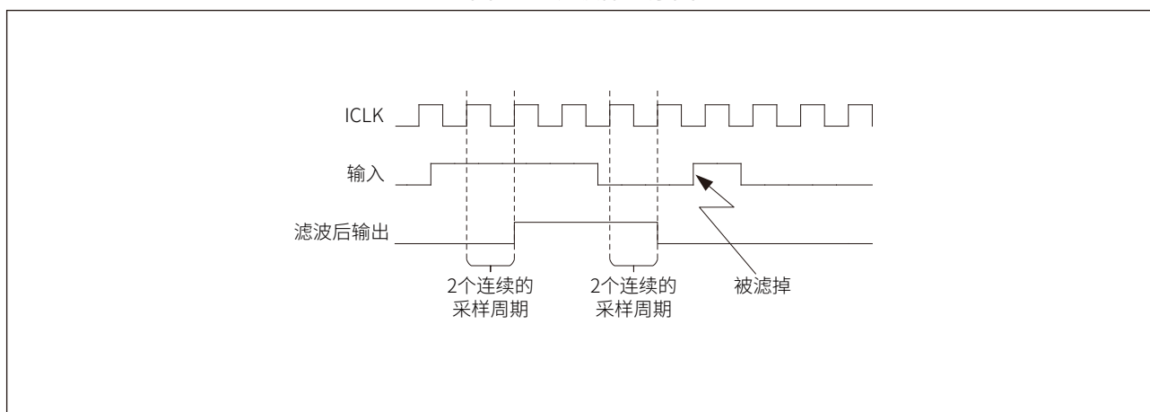
图 15-2 滤波器时序图
