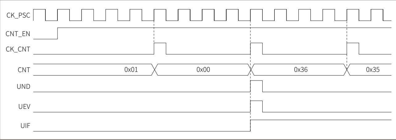
图 16-11 递减计数，内部时钟分频因子为 4
