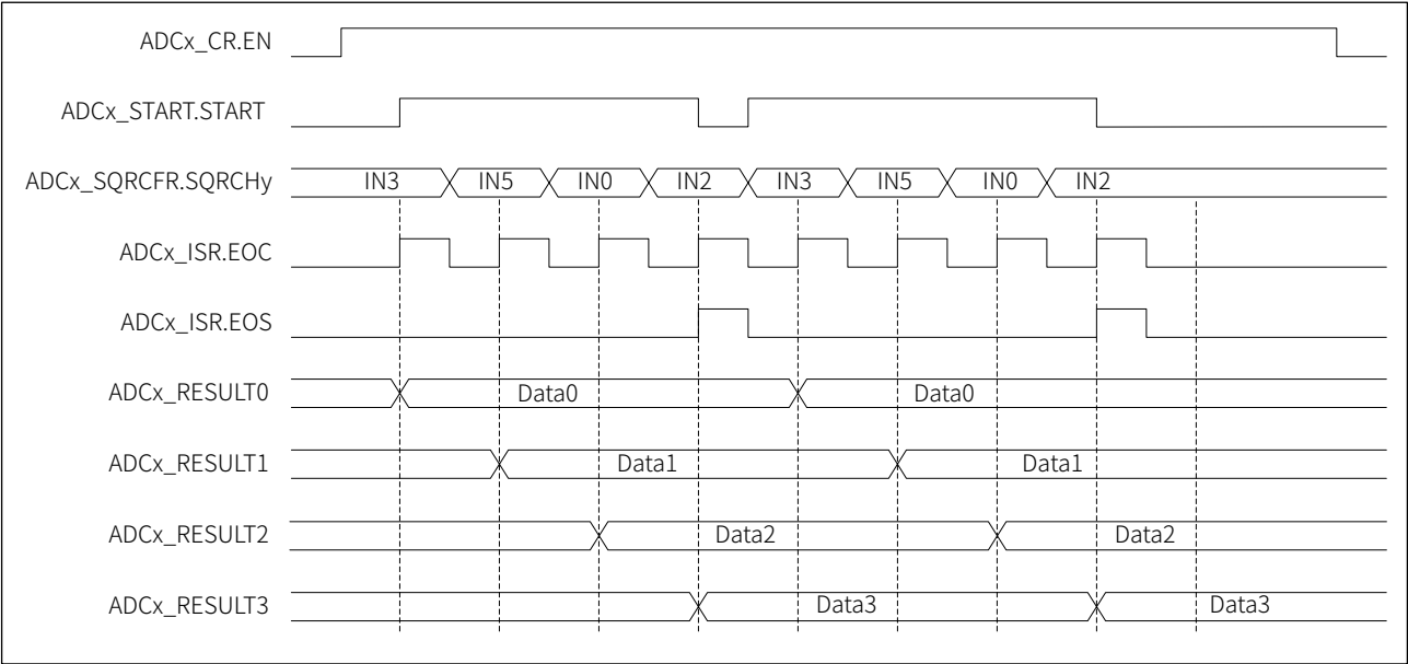
图 25-4 序列扫描转换时序图
