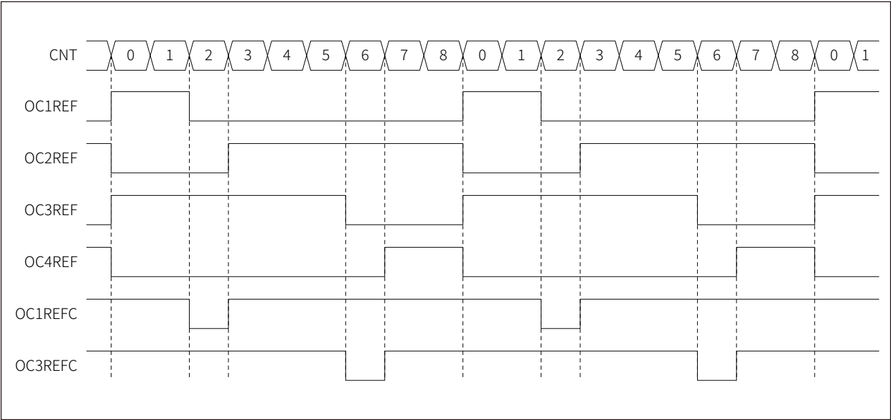
图 17-42 组合 PWM 模式 1 示例
