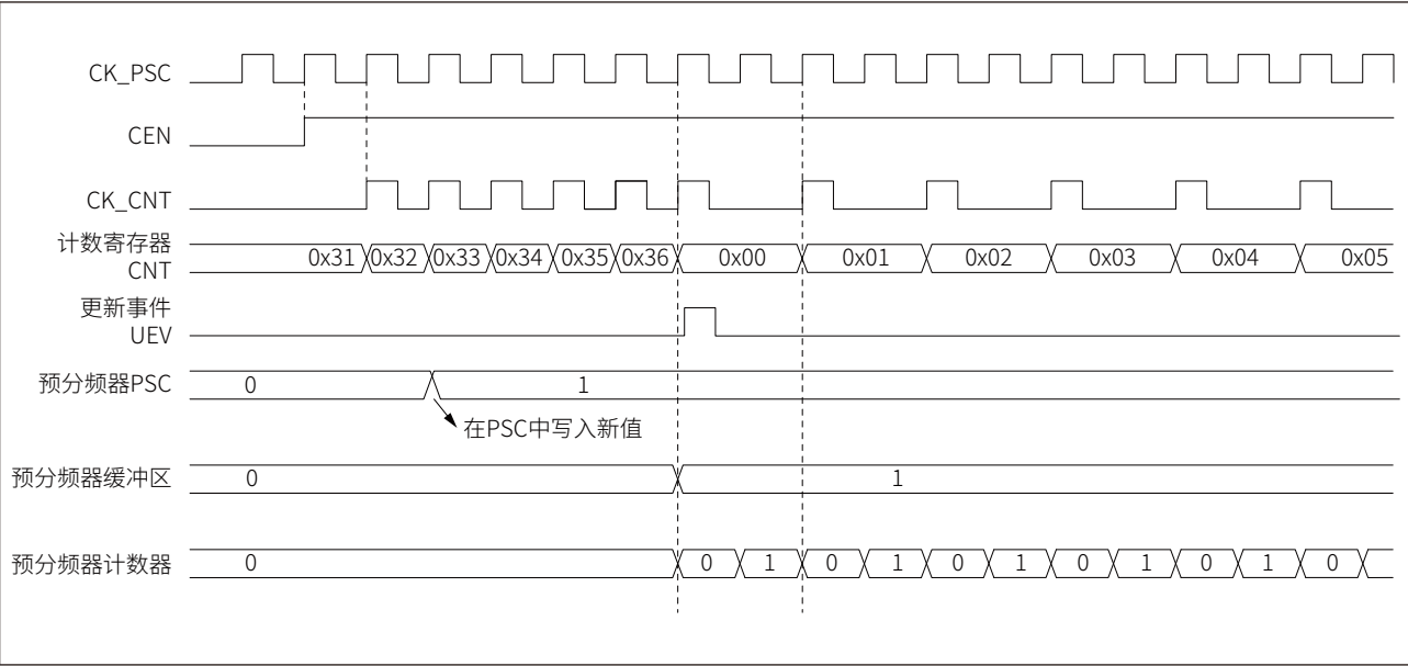
图 17-2 预分频器分频由 1 变为 2 时的时序图
