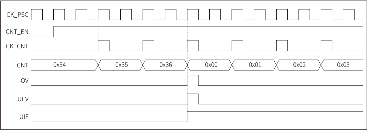
图 17-5 递增计数，内部时钟分频因子为 4
