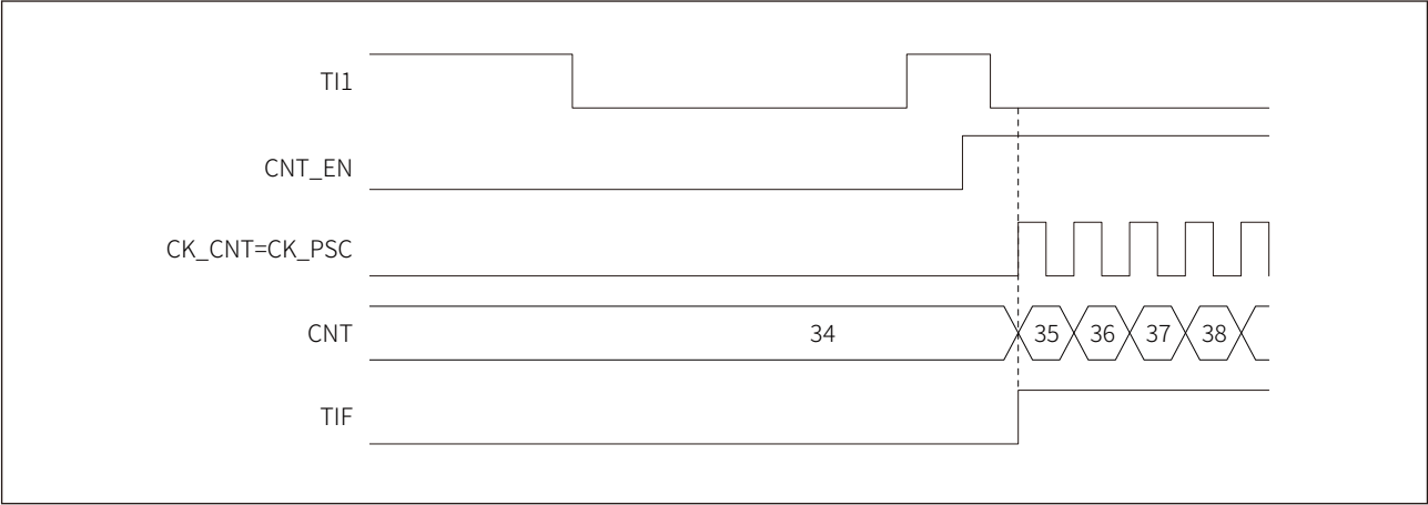
图 17-27 触发模式时序
