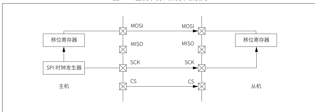
图 22-8 主机单发、从机单收模式
