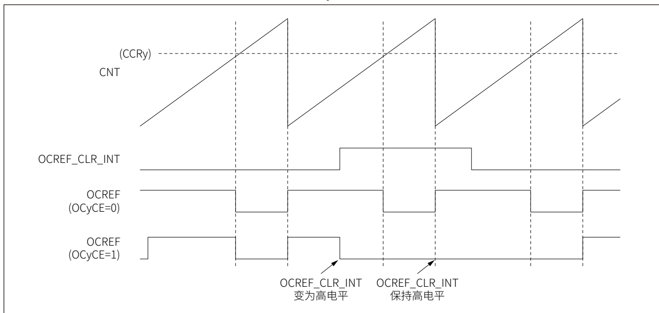
图 17-53 OCyREF 清零示例
