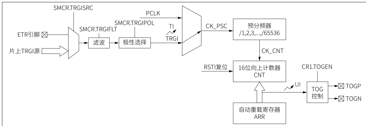
图 14-6 外部计数模式框图
