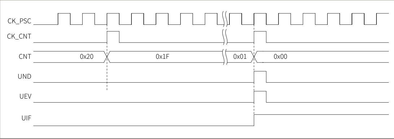
图 17-16 中心对齐模式，内部时钟分频因子为 N
