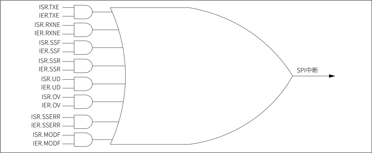
图 22-11 SPI 中断
