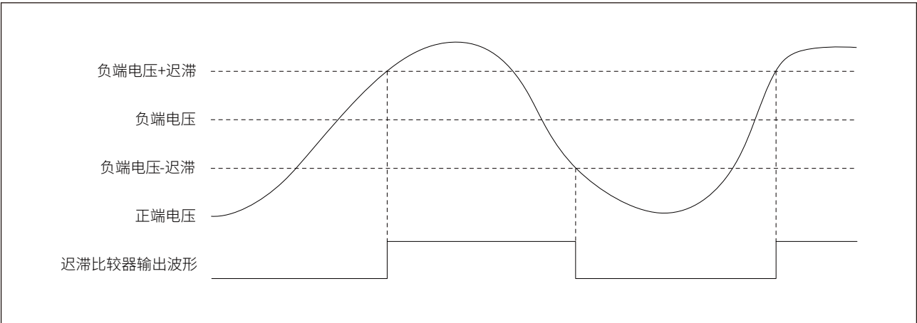
图 27-3 VC 迟滞功能
