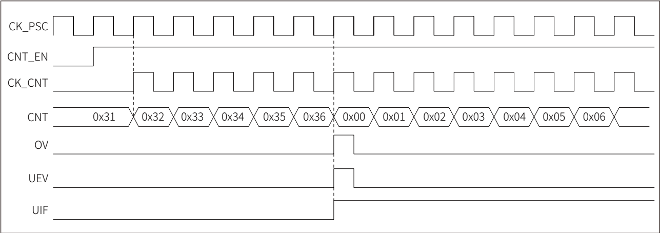
图 17-3 递增计数，内部时钟分频因子为 1
