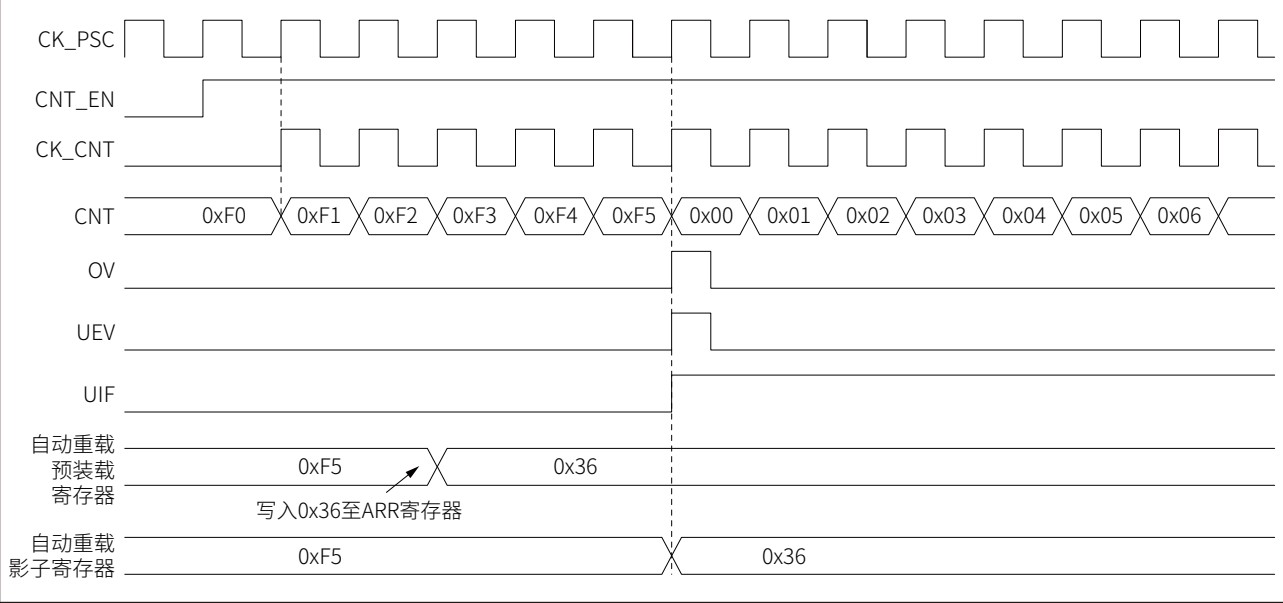
图 17-8 递增计数，当重载缓存使能时的更新事件 (ATIM_CR1.ARPE=1)
