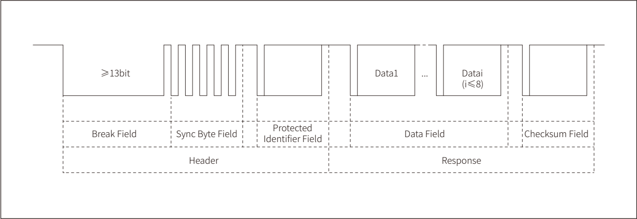
图 21-12 LIN 帧的结构
