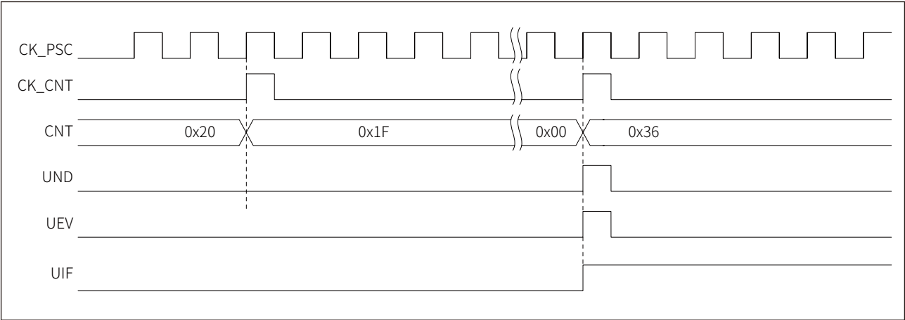
图 16-12 递减计数，内部时钟分频因子为 N
