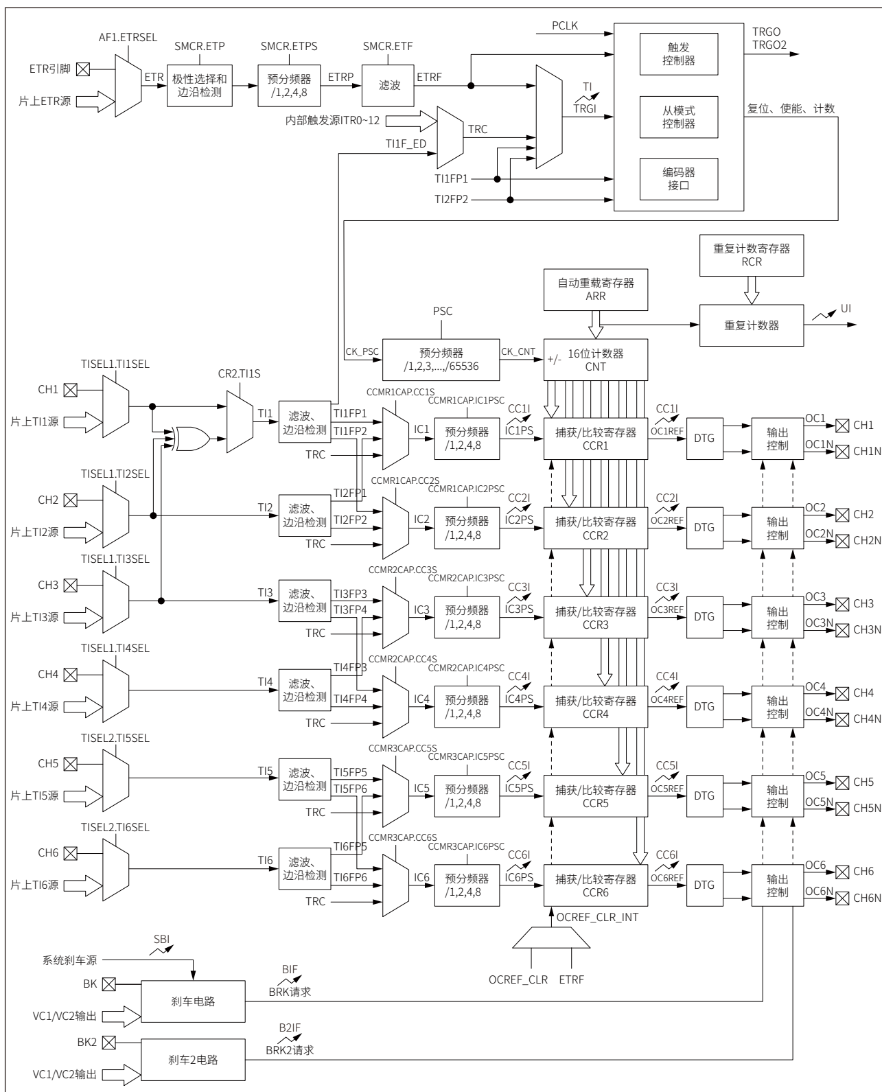
图 17-1 ATIM 功能框图
