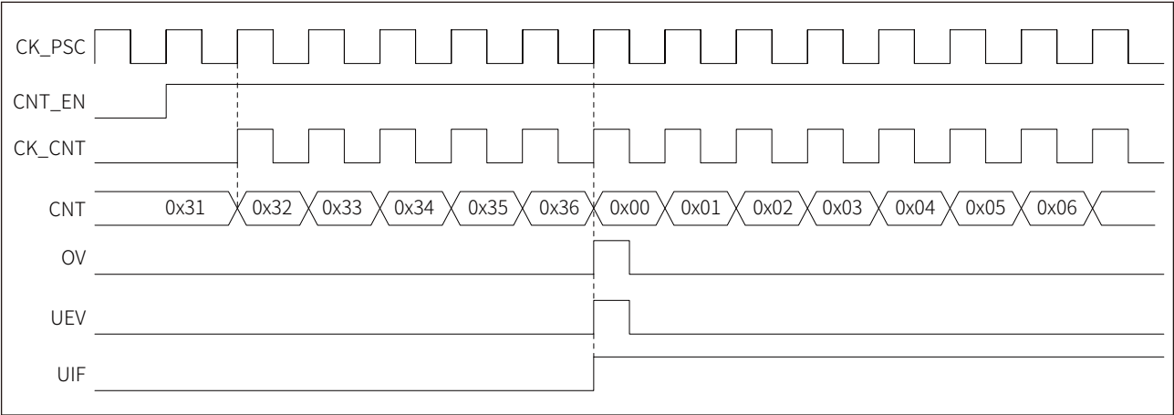
图 16-3 递增计数，内部时钟分频因子为 1
