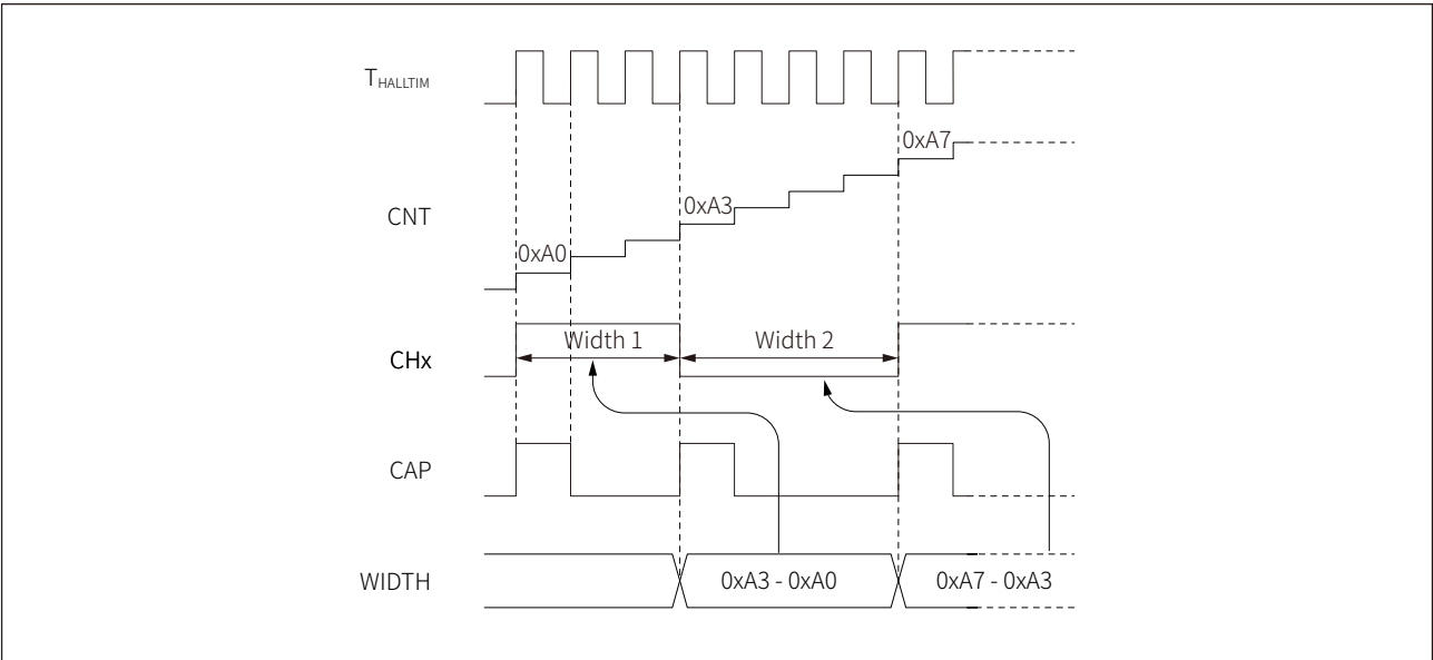
图 18-2 输入捕获模式框图
