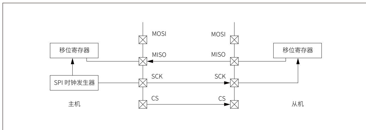
图 22-9 主机单收、从机单发模式
