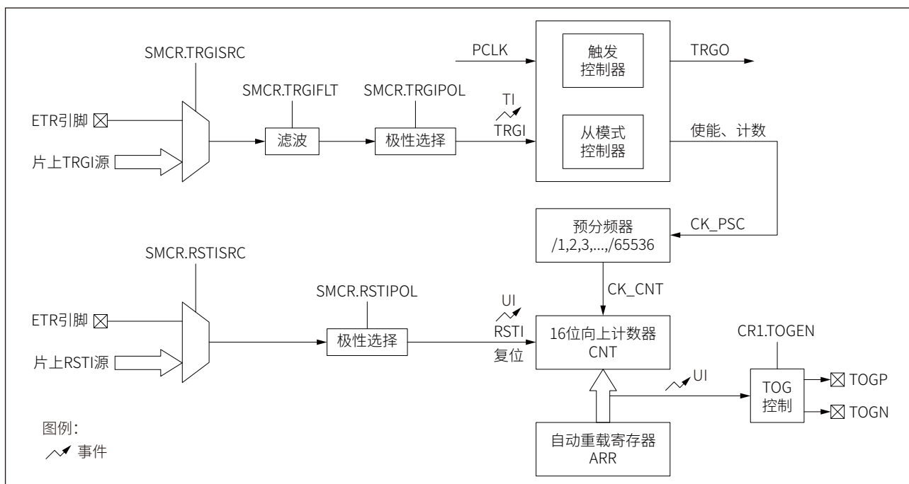
图 14-1 BTIM 功能框图
