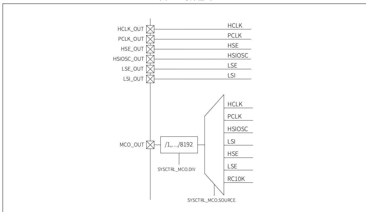
图 4-5 时钟输出
