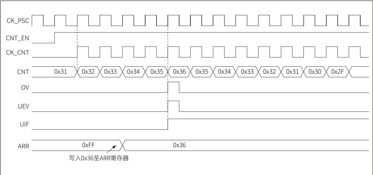
图 16-18 中心对齐模式，当重载缓存使能时的更新事件 (GTIMx_CR1.ARPE=1)
