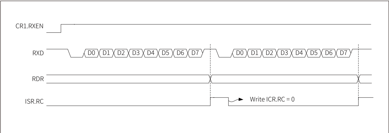
图 21-6 异步工作模式接收控制时序（接收两个字节数据）
