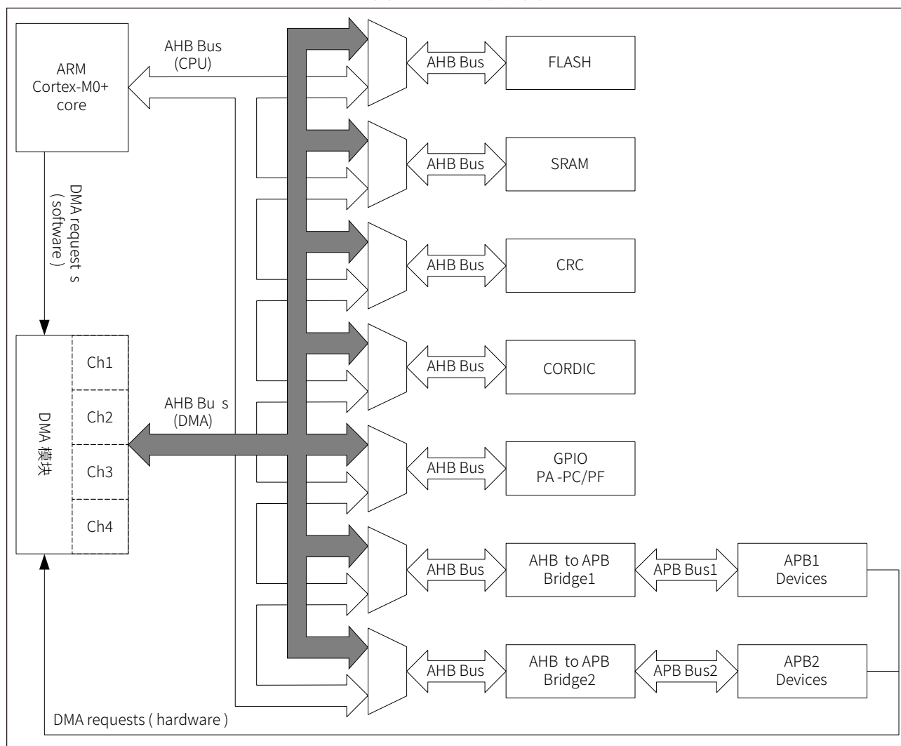
图 8-1 DMA 功能框图
