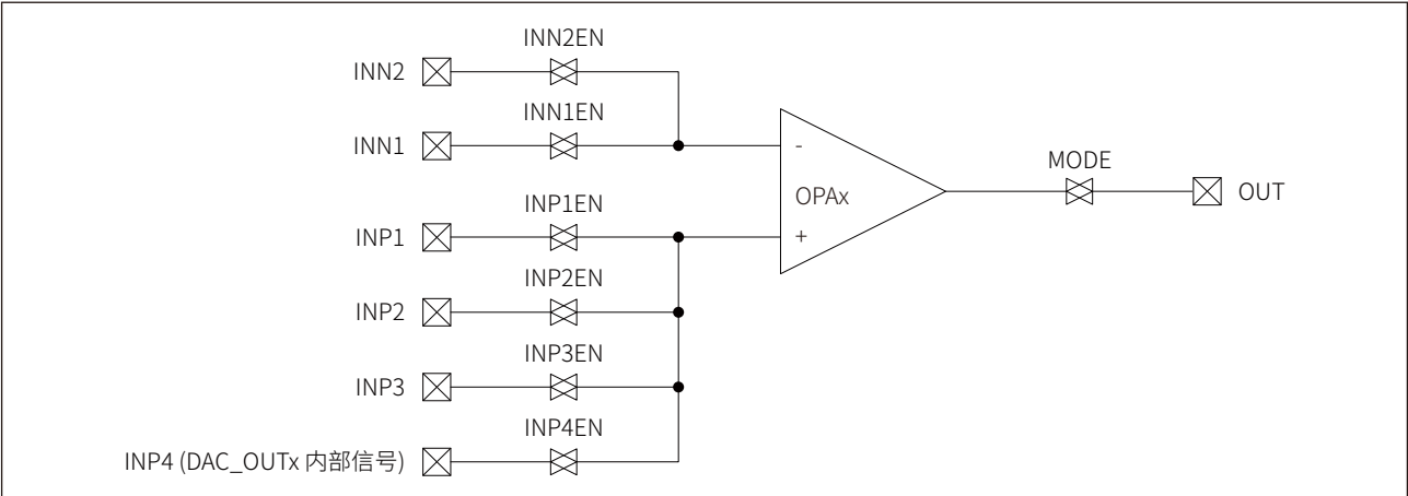
图 29-1 OPA功能框图
