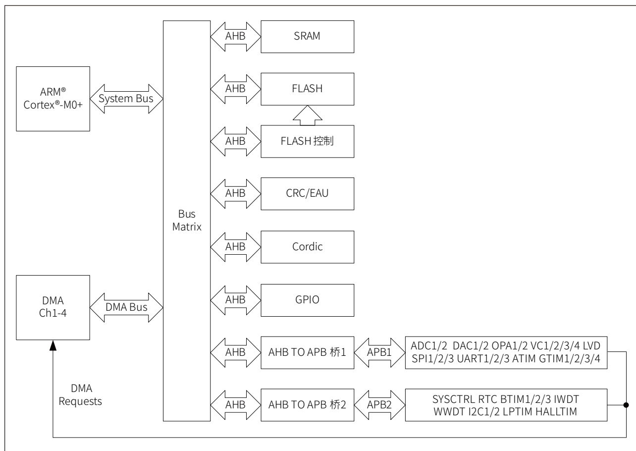
图 2-1 系统架构
