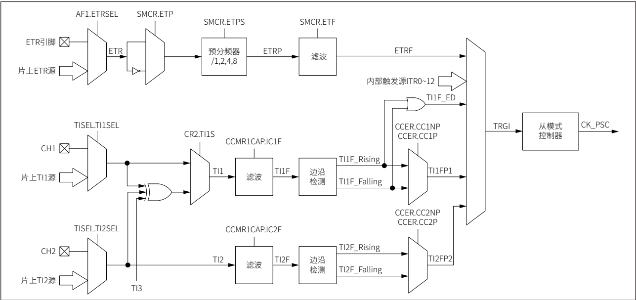
图 16-21 外部时钟模式 1 连接图
