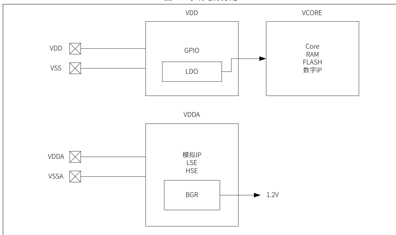
图 3-1 系统电源分配
