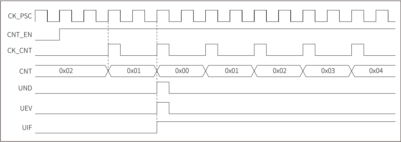
图 16-15 中心对齐模式，内部时钟分频因子为 4，ARR=0x36
