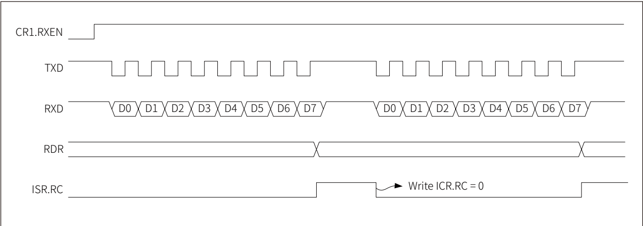
图 21-3 同步半双工模式接收时序（接收两个字节数据）
