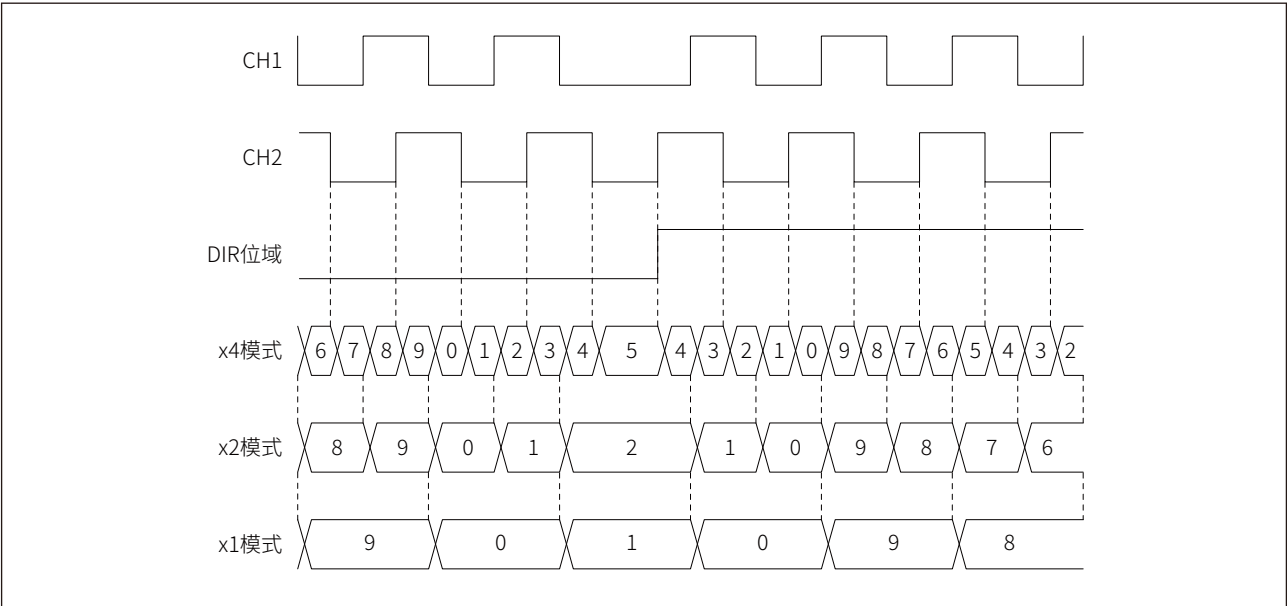
图 17-30 各正交编码器模式计数示例
