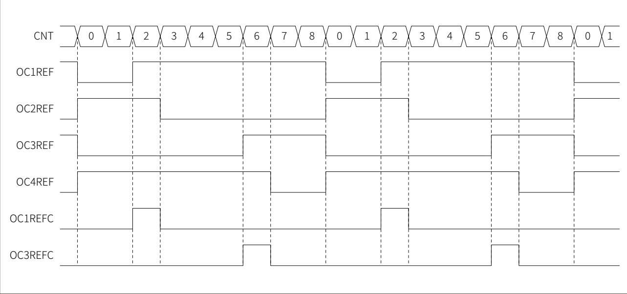
图 16-43 组合 PWM 模式 2 示例
