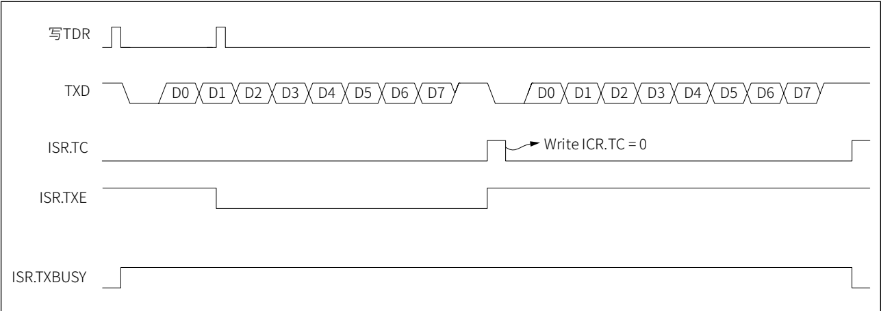
图 21-4 异步工作模式发送控制时序（发送两个字节数据）
