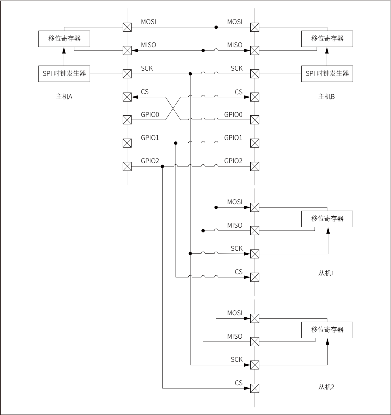
图 22-10 多机通信系统
