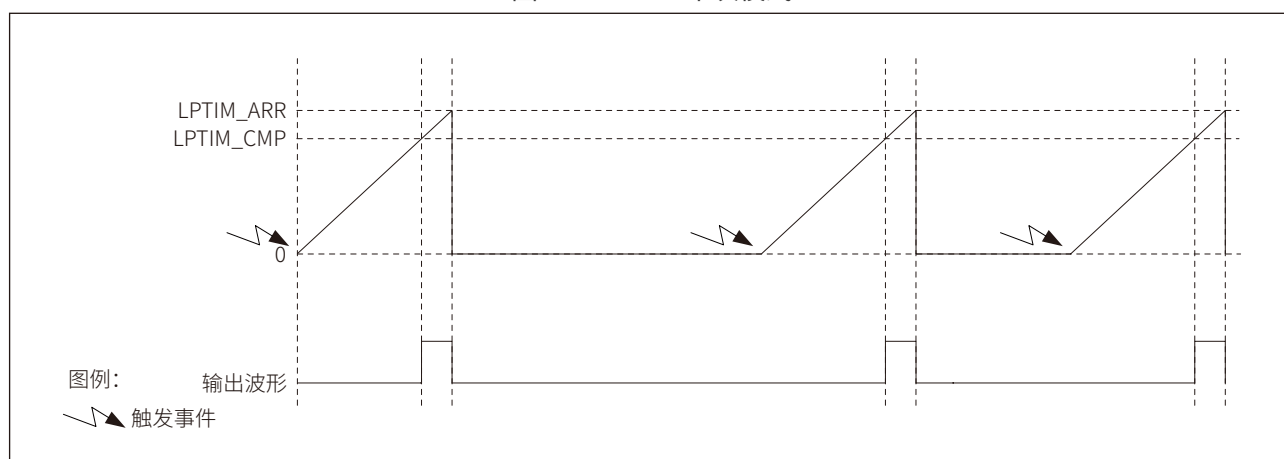
图 15-3 LPTIM 单次模式
