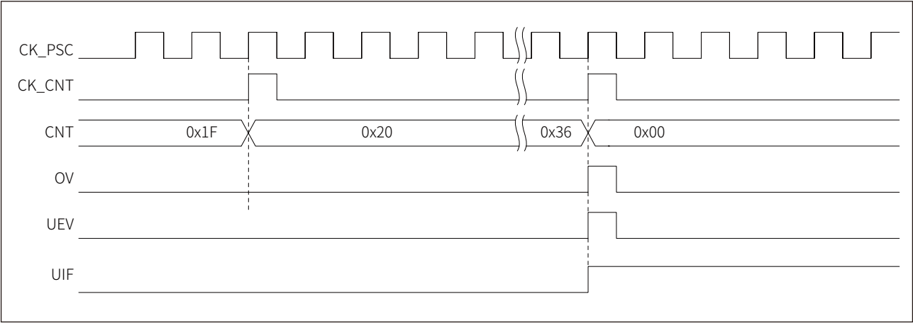
图 17-6 递增计数，内部时钟分频因子为 N
