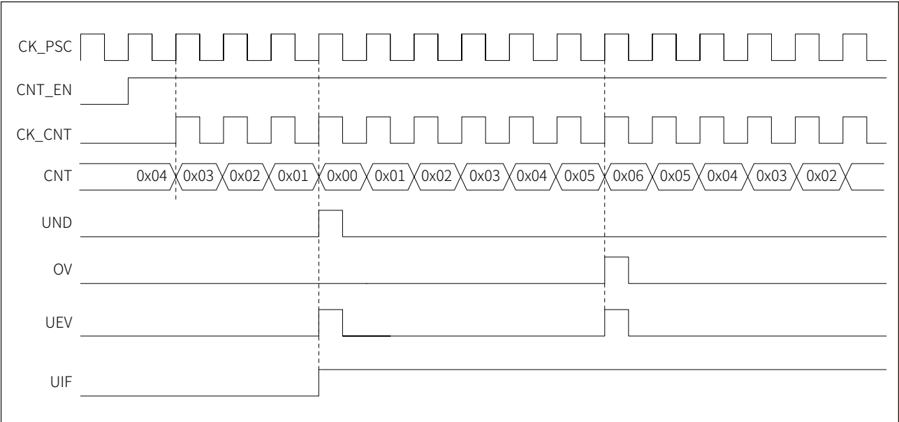
图 16-13 中心对齐模式，内部时钟分频因子为 1，ARR=0x06
