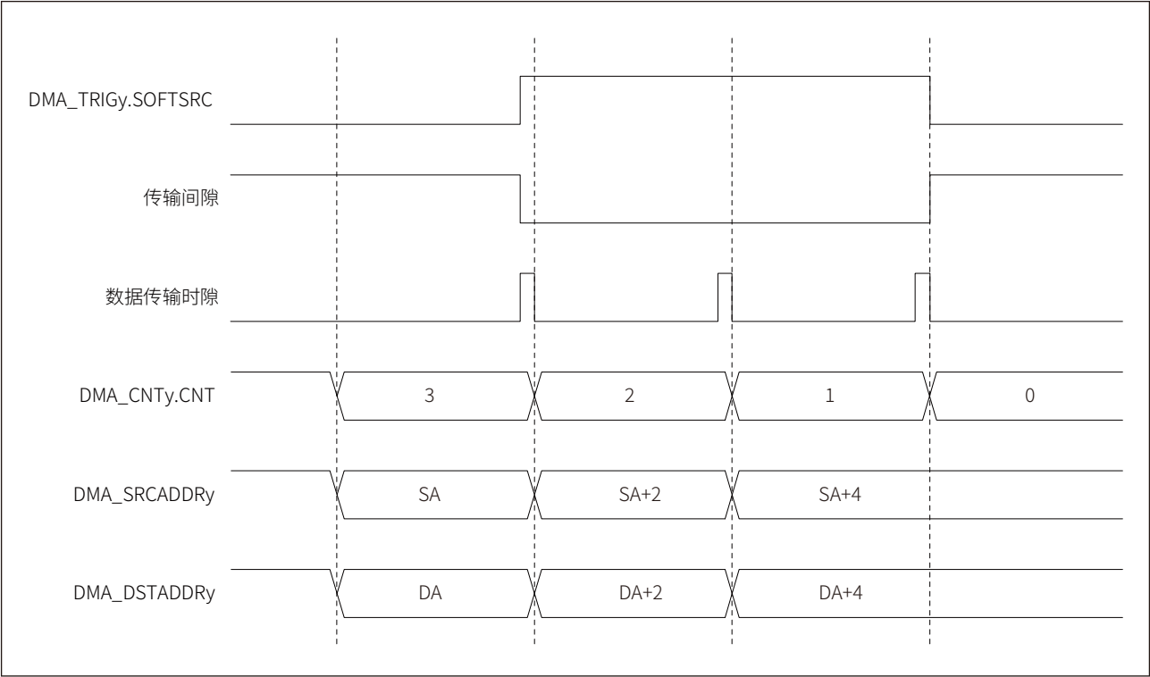
图 8-3 软件触发BULK传输模式
