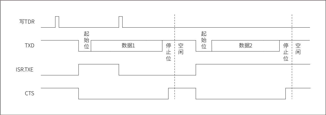
图 21-9 CTS 流控时序
