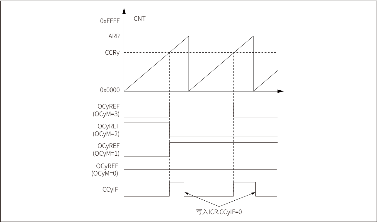
图 16-36 比较匹配输出模式
