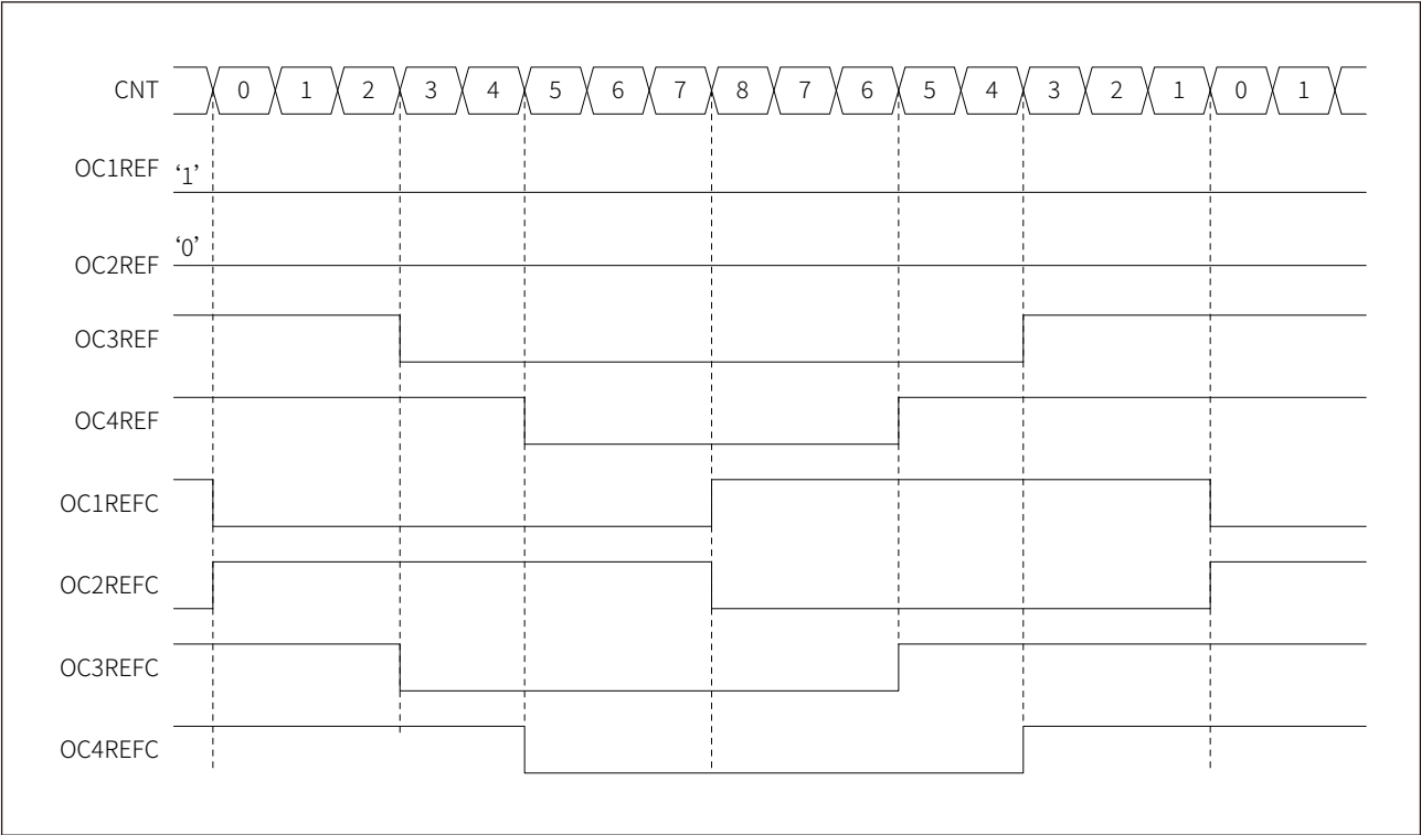
图 16-40 不对称 PWM 模式 1 示例
