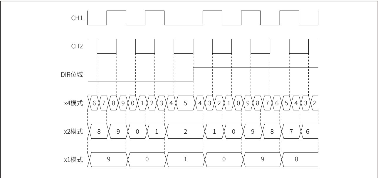
图 16-29 各正交编码器模式计数示例
