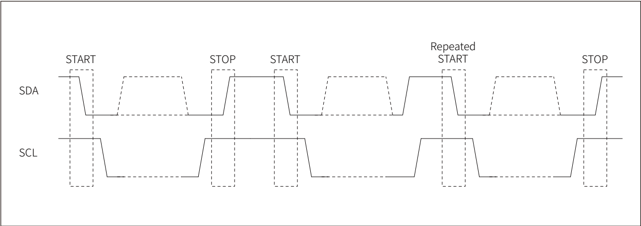
图 23-2 起始和停止信号
