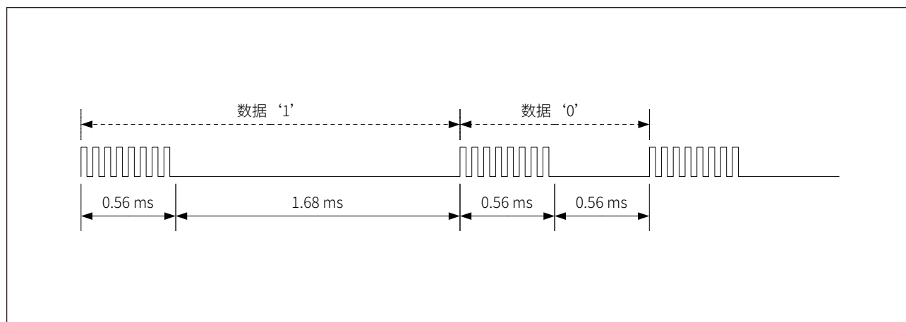
图 24-1 PWM 调制方式
