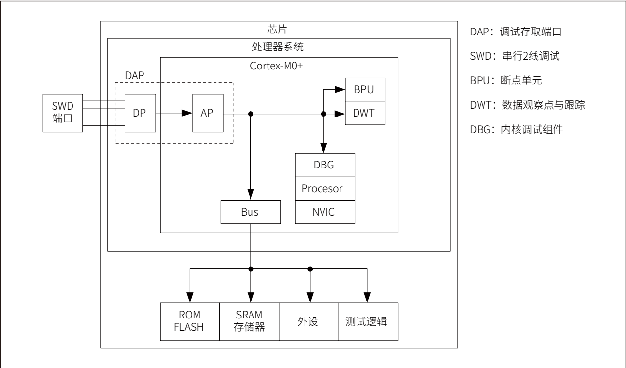
图 30-1 SWD 功能框图
