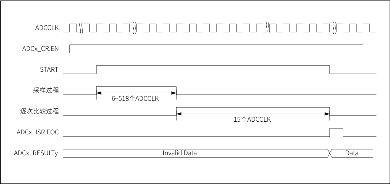
图 25-2 ADC 转换时序图
