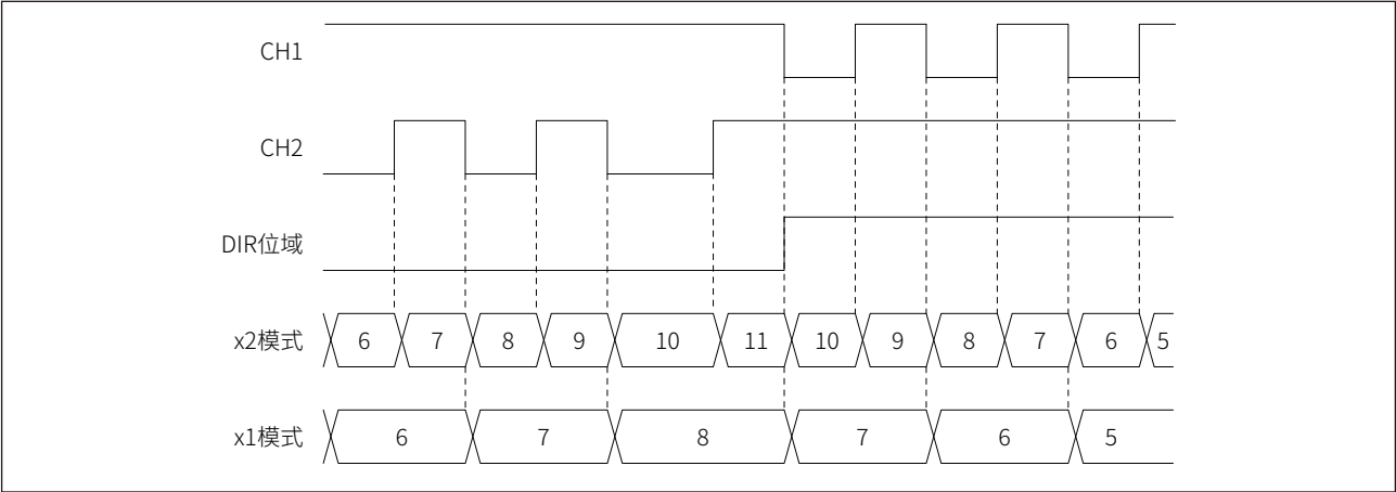
图 16-32 定向时钟编码器模式计数示例 (CC1P = CC2P = 1)
