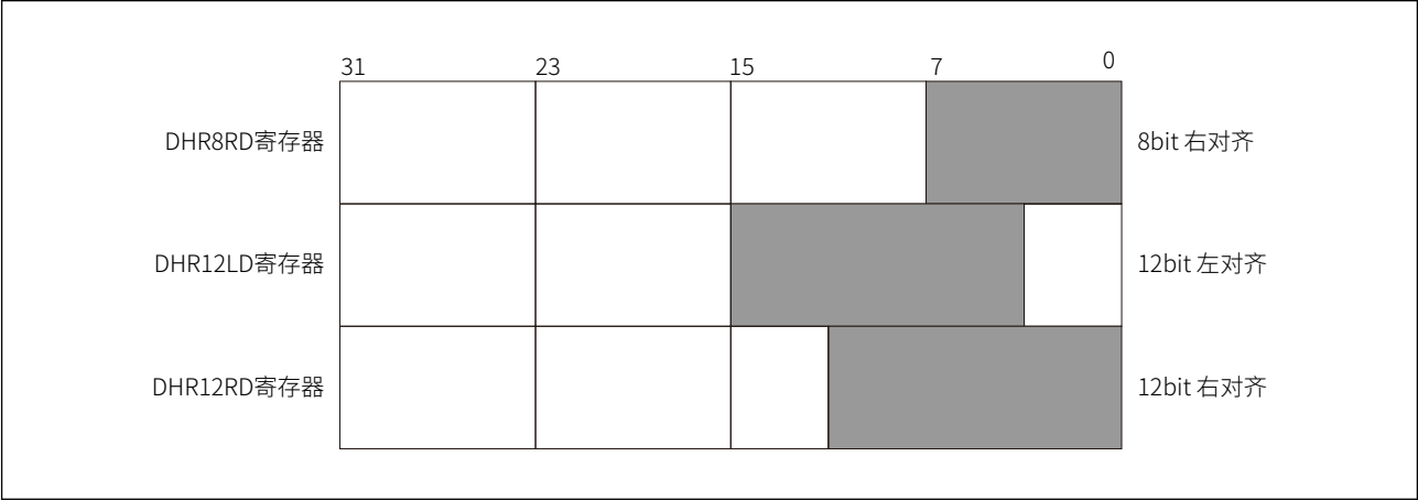
图 26-2 单通道寄存器配置格式
