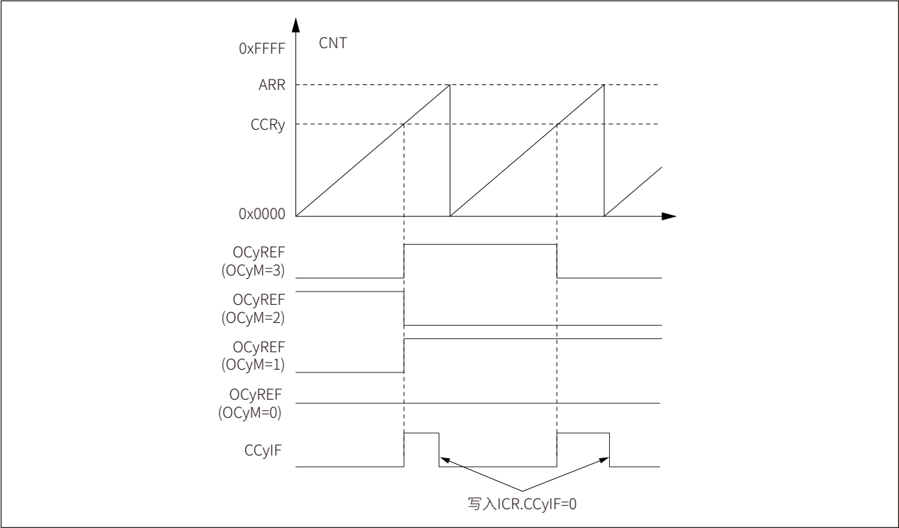
图 17-36 比较匹配输出模式
