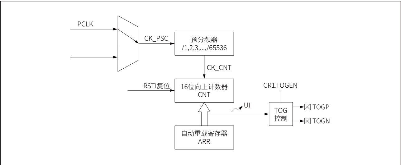
图 14-5 内部计数模式框图
