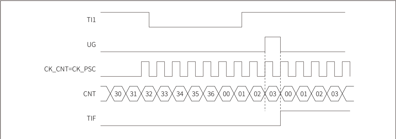
图 16-24 复位模式时序
