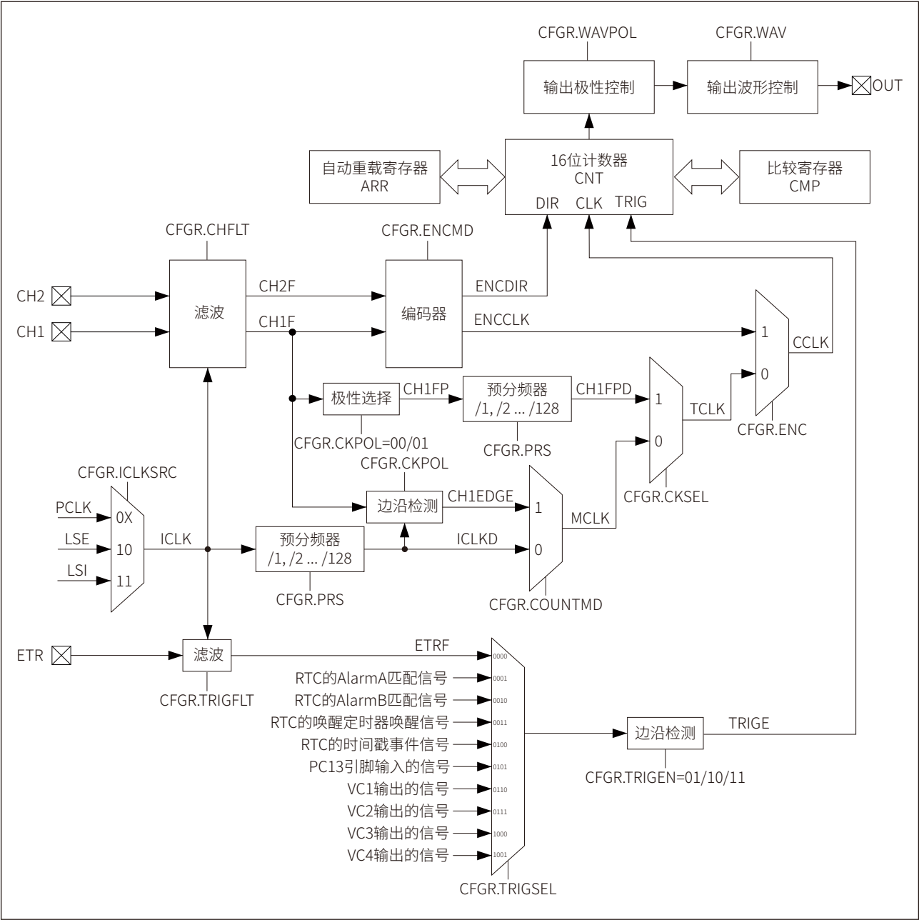
图 15-1 LPTIM功能框图
