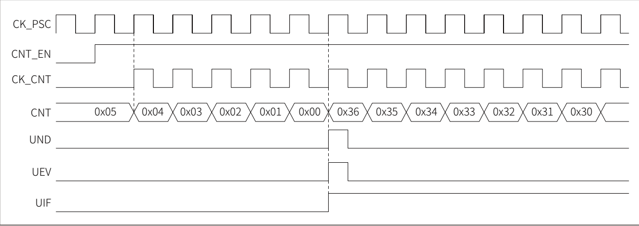
图 16-10 递减计数，内部时钟分频因子为 2
