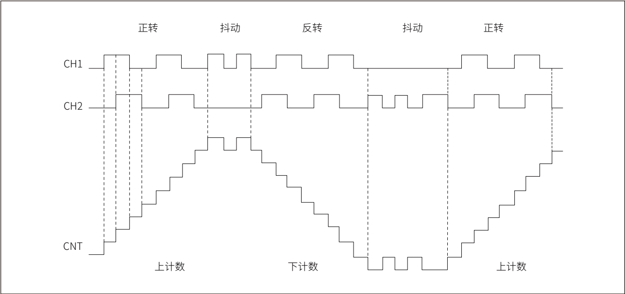
图 17-29 正交编码器模式-x4 模式操作示例
