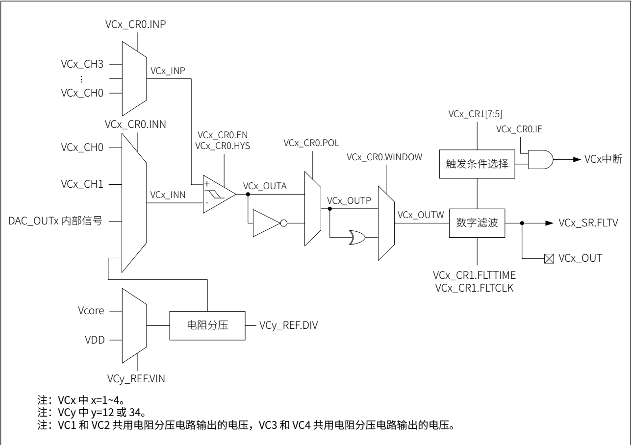
图 27-1 VC 功能框图
