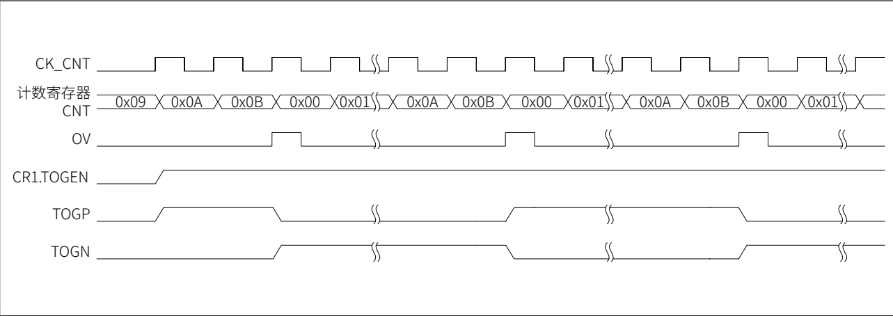
图 14-4 电平翻转输出示意图（ARR=0x0B）
