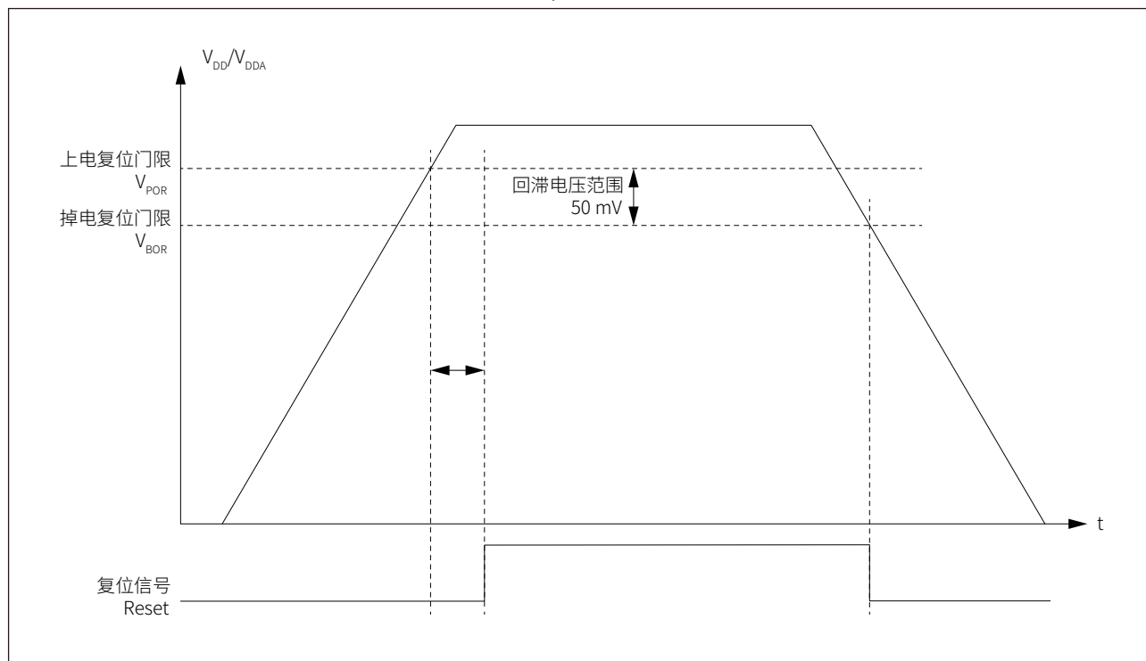
图 3-2 上电/掉电复位时序图
