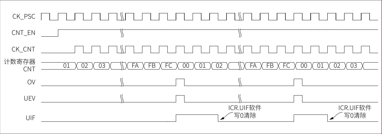
图 14-3 连续计数模式示例
