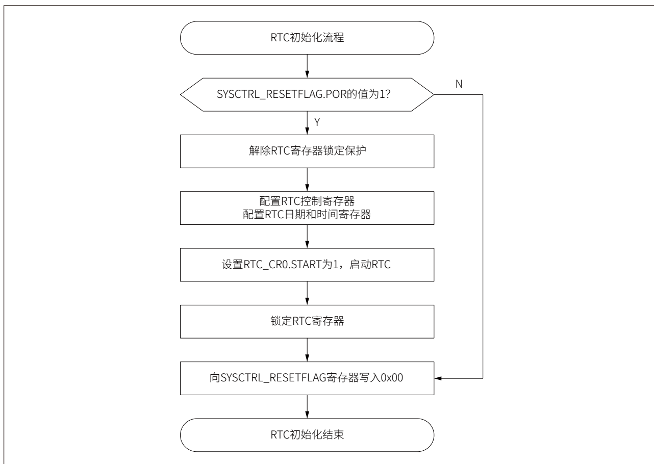
图 13-2 RTC 初始化流程
