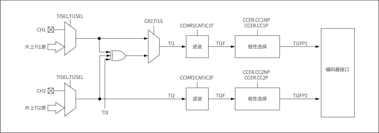
图 16-27 编码器模式框图
