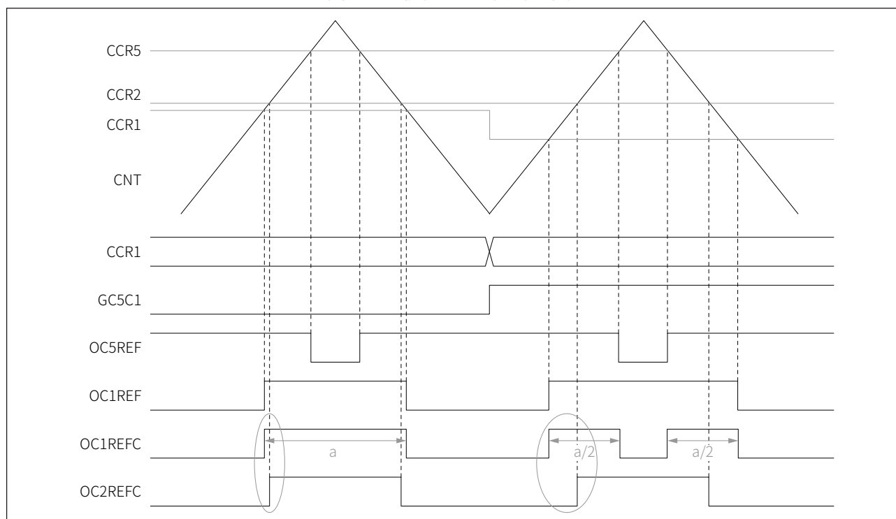
图 17-44 移相 PWM 模式 5 示例
