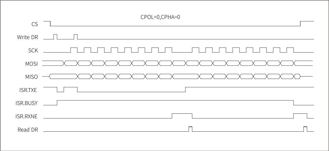
图 22-5 全双工模式下主机收发时序（两个字节）
