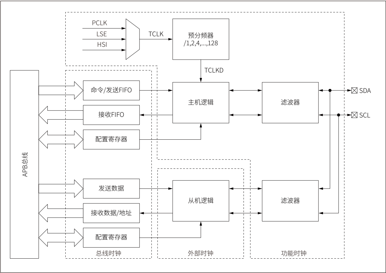
图 23-6 I2C 功能框图
