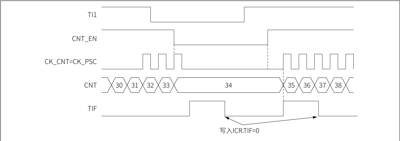
图 16-25 门控模式时序
