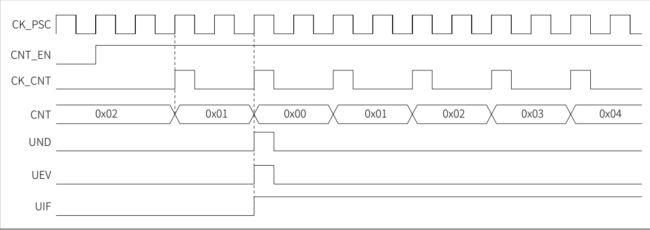
图 17-15 中心对齐模式，内部时钟分频因子为 4，ARR=0x36
