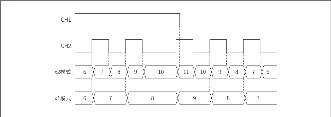
图 17-31 时钟加方向编码器模式计数示例
