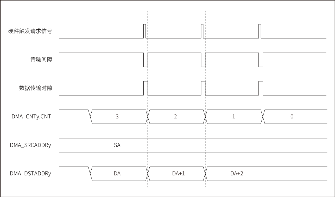
图 8-4 硬件触发 BLOCK 传输模式
