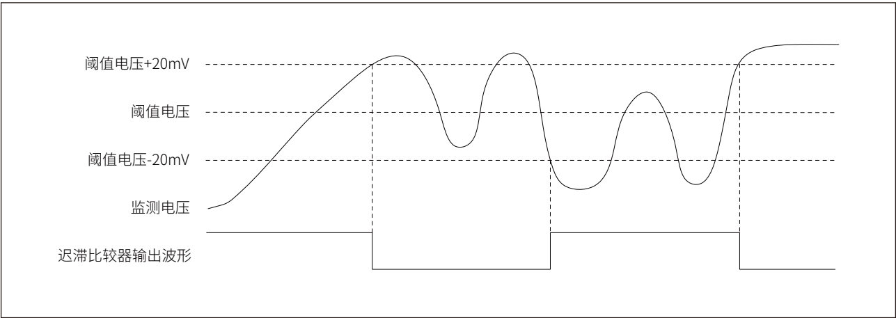
图 28-2 LVD 迟滞响应
