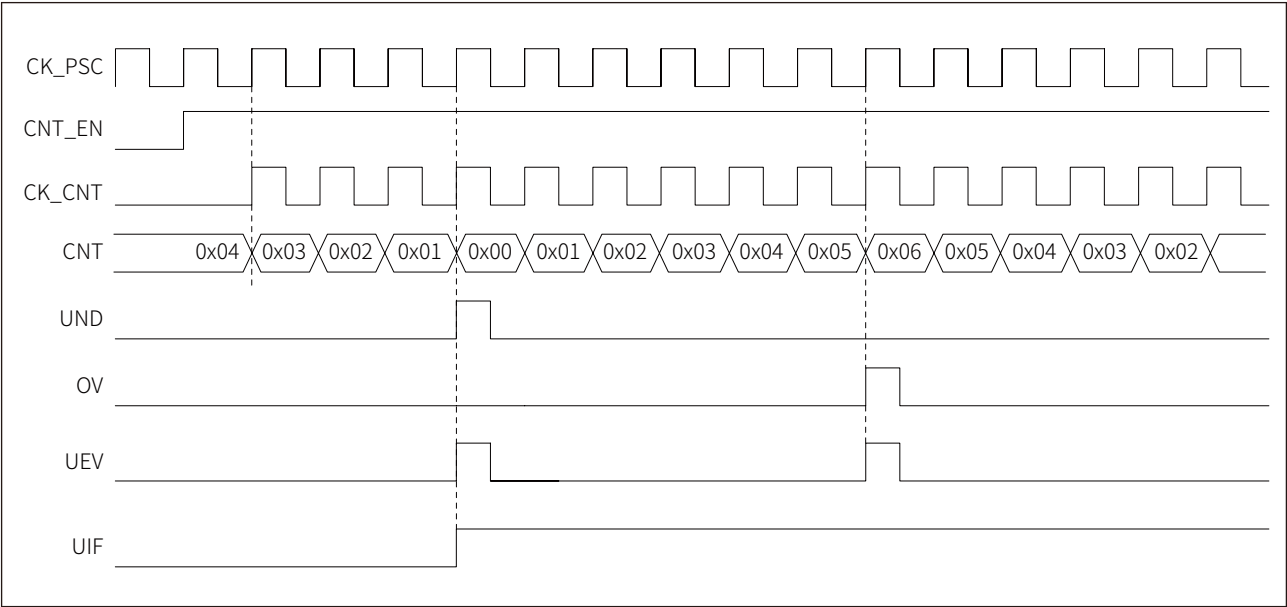
图 17-13 中心对齐模式，内部时钟分频因子为 1，ARR=0x06
