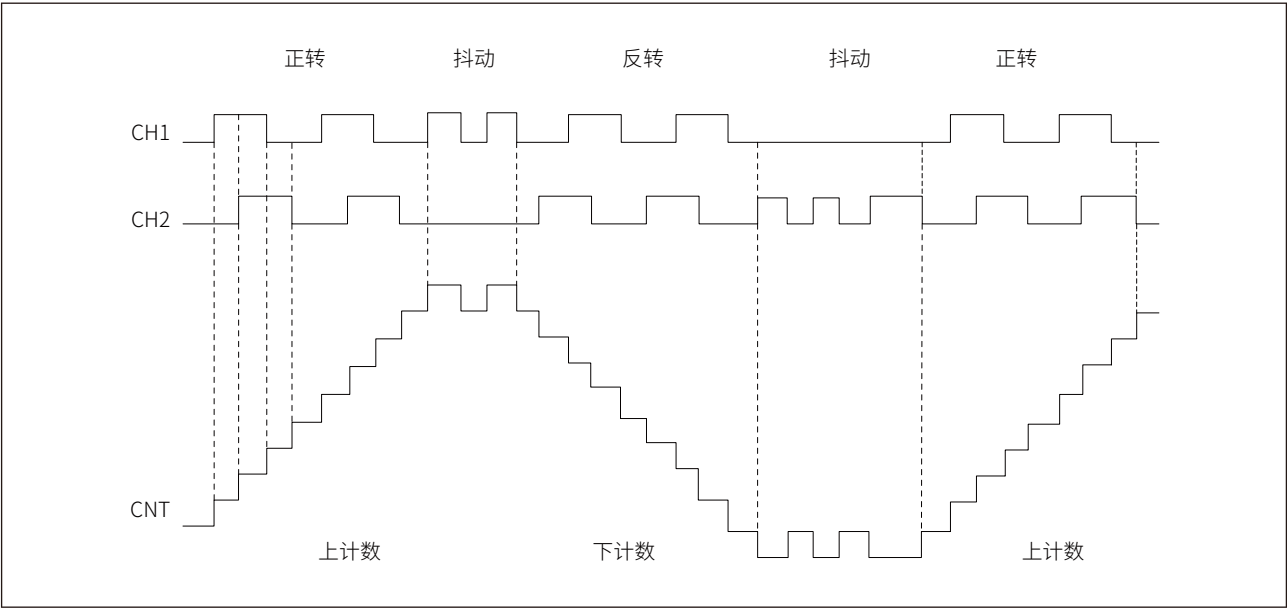
图 16-28 正交编码器模式-x4 模式操作示例
