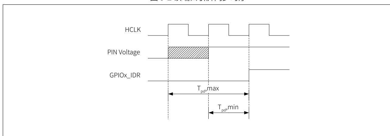
图 9-2 读端口引脚同步时序
