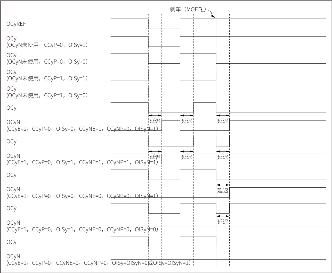
图 17-50 响应刹车事件 BRK 时的输出行为 (OSSI=0)
