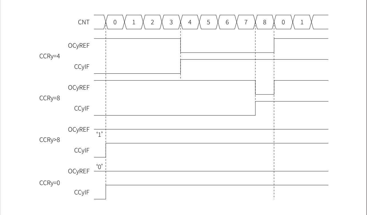
图 16-37 PWM 模式 1，边沿对齐模式，递增计数
