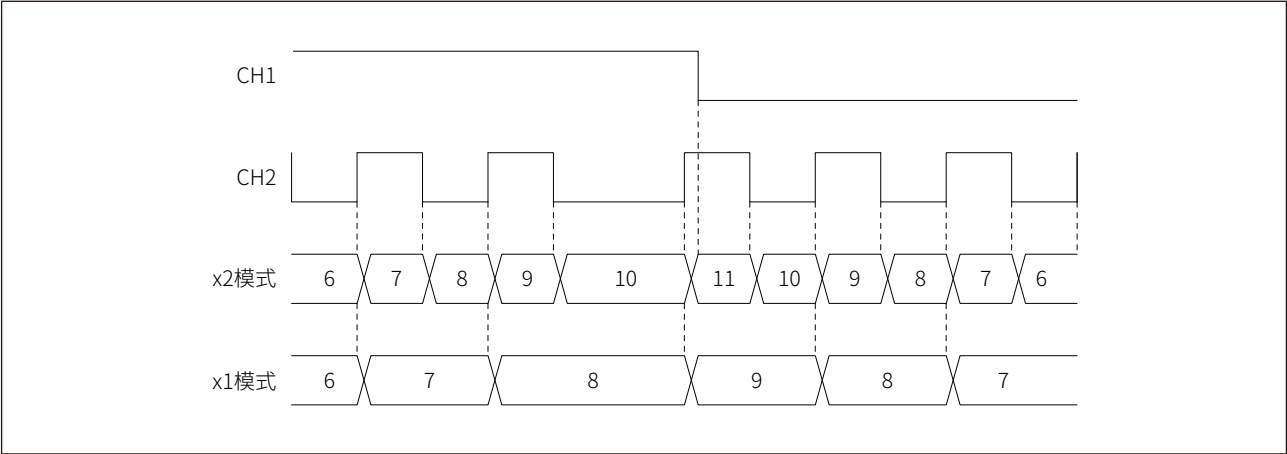
图 16-30 时钟加方向编码器模式计数示例
