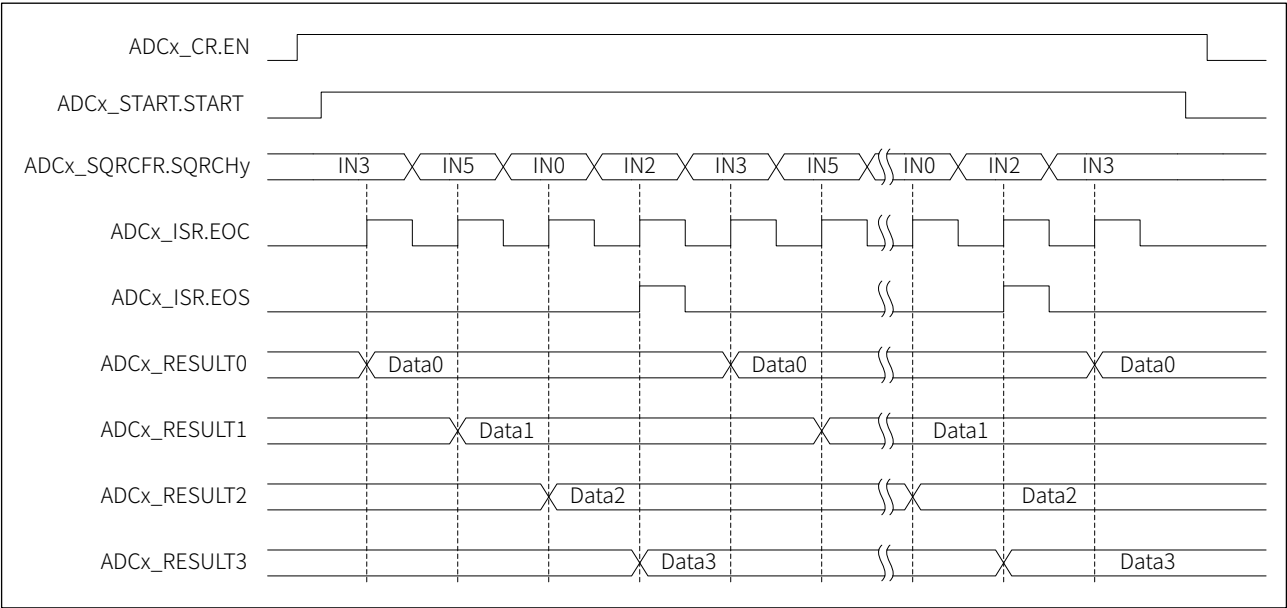
图 25-3 序列连续转换时序图
