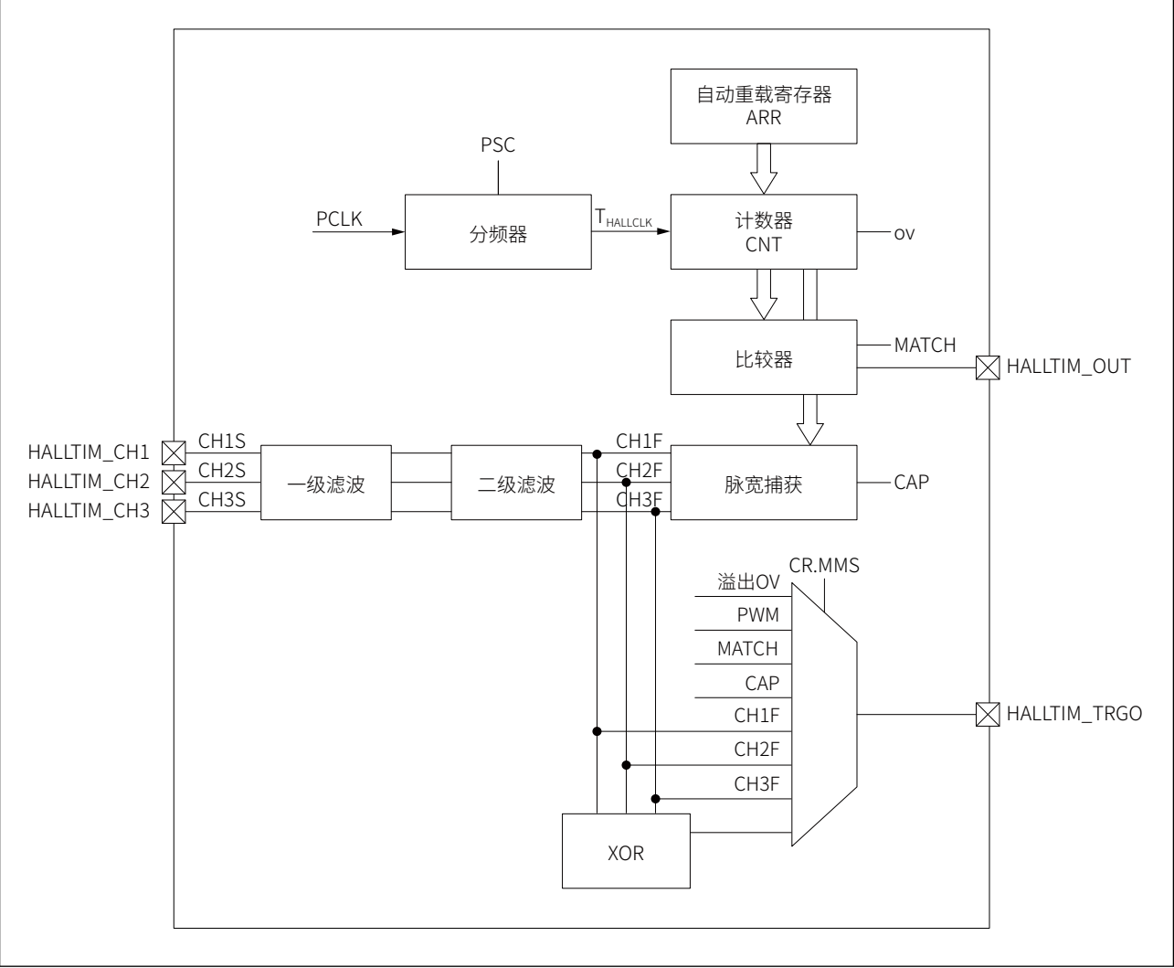
图 18-1 HALLTIM 功能框图
