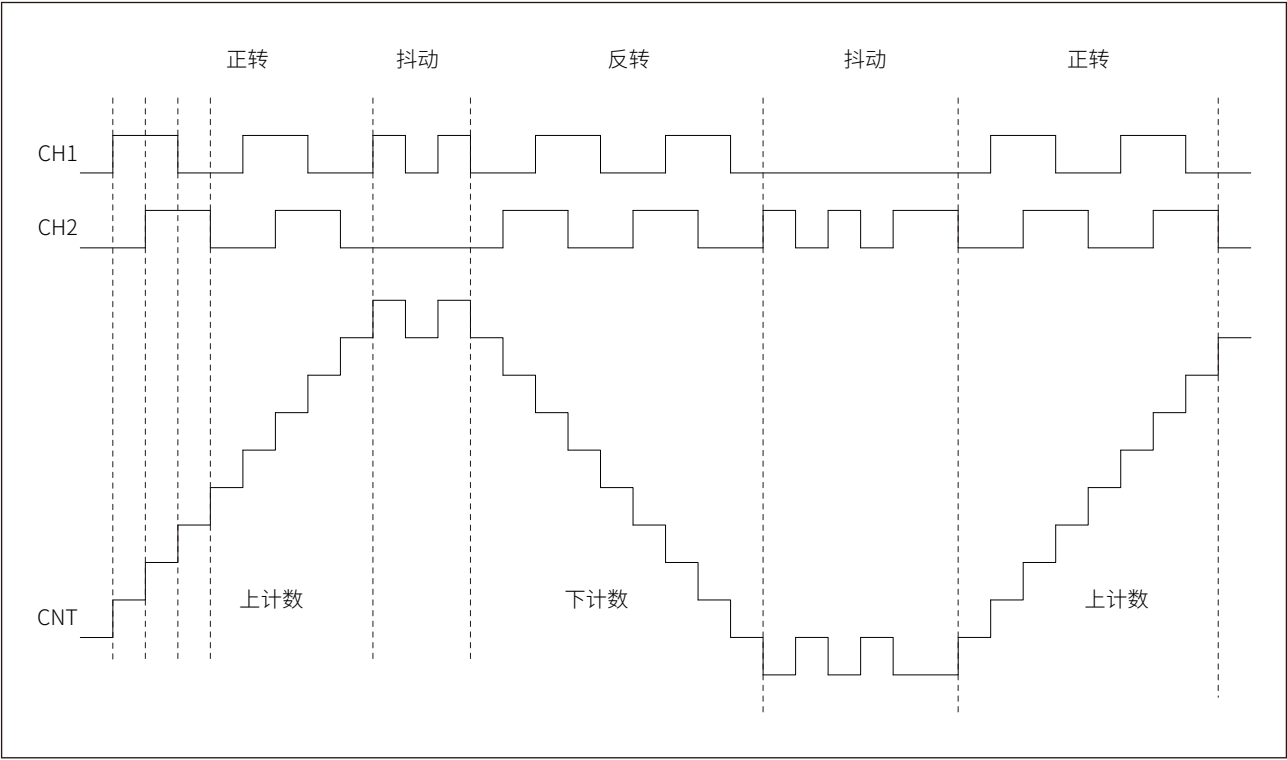
图 15-7 编码器模式计数示例
