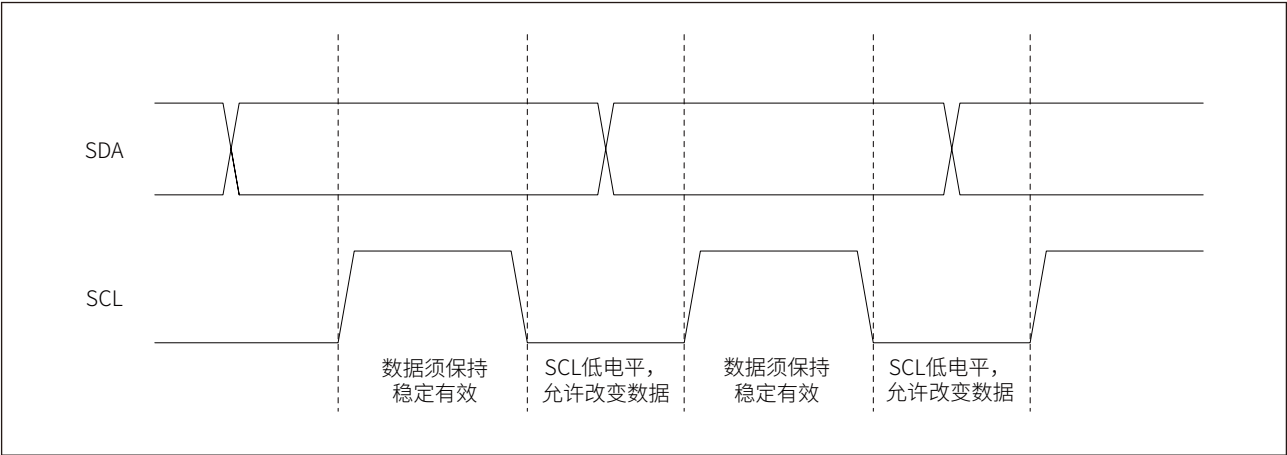
图 23-3 数据传输
