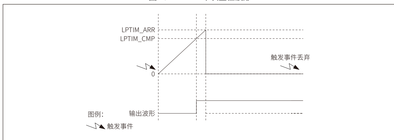
图 15-4 LPTIM 单次置位波形
