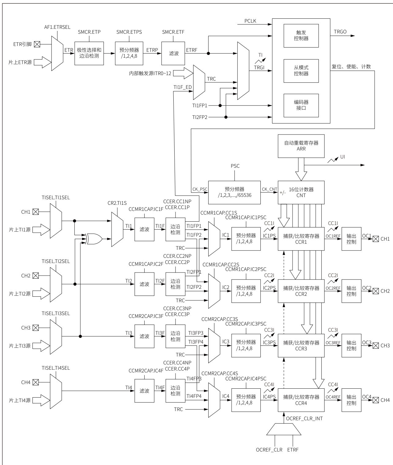
图 16-1 GTIM 功能框图
