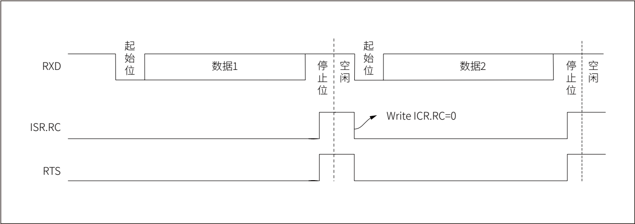
图 21-8 RTS 流控时序
