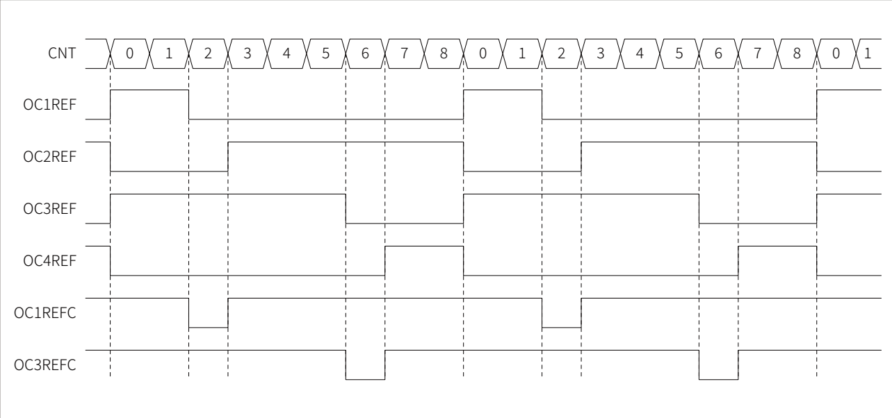
图 16-42 组合 PWM 模式 1 示例
