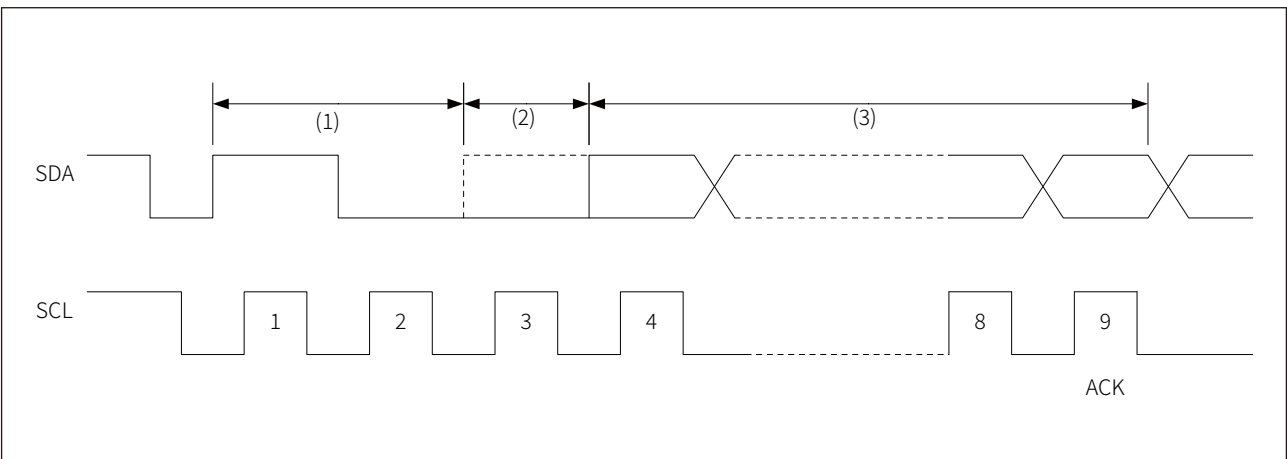
图 23-5 冲突检测及仲裁
