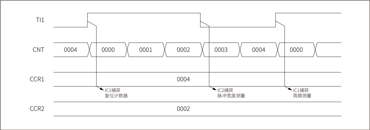
图 17-35 PWM 输入模式时序
