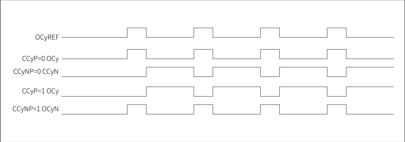
图 17-46 互补 PWM 输出波形
