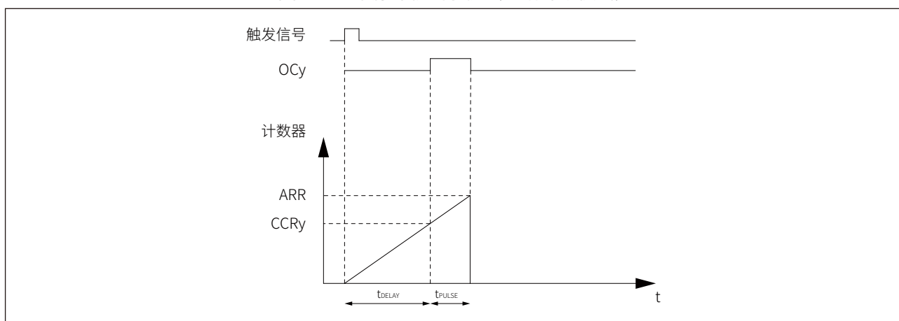
图 17-20 单脉冲输出示例（递增计数模式）
