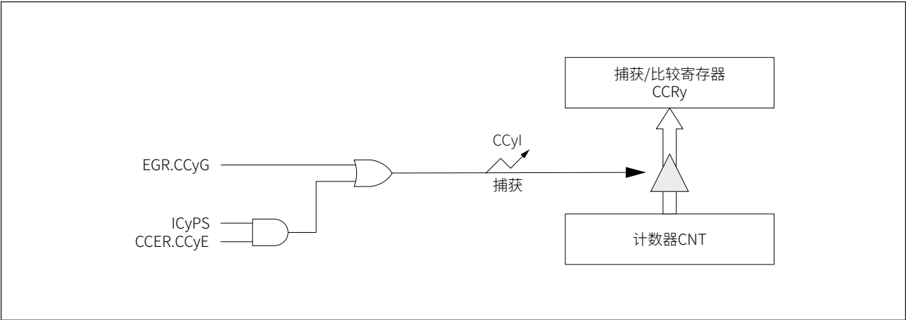
图 17-34 输入捕获模式框图
